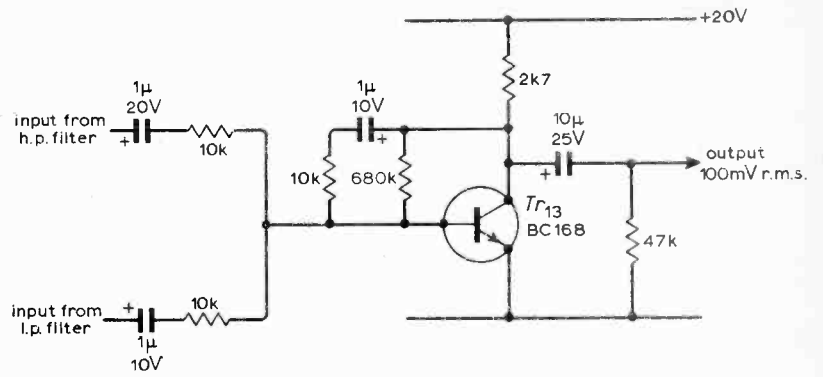
Fig. 18. Adding amplifier.
