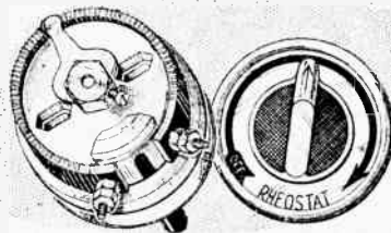
Igranic Pacent filament rheostat.
