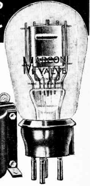
Marconi D E 5 (6 volt) 22/6
