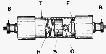
Permanent carborundum detector (No. 251,078.)
