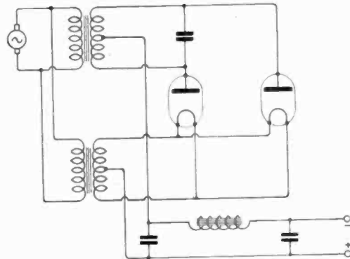
Fig. 5. Circuit of Rectifier.
