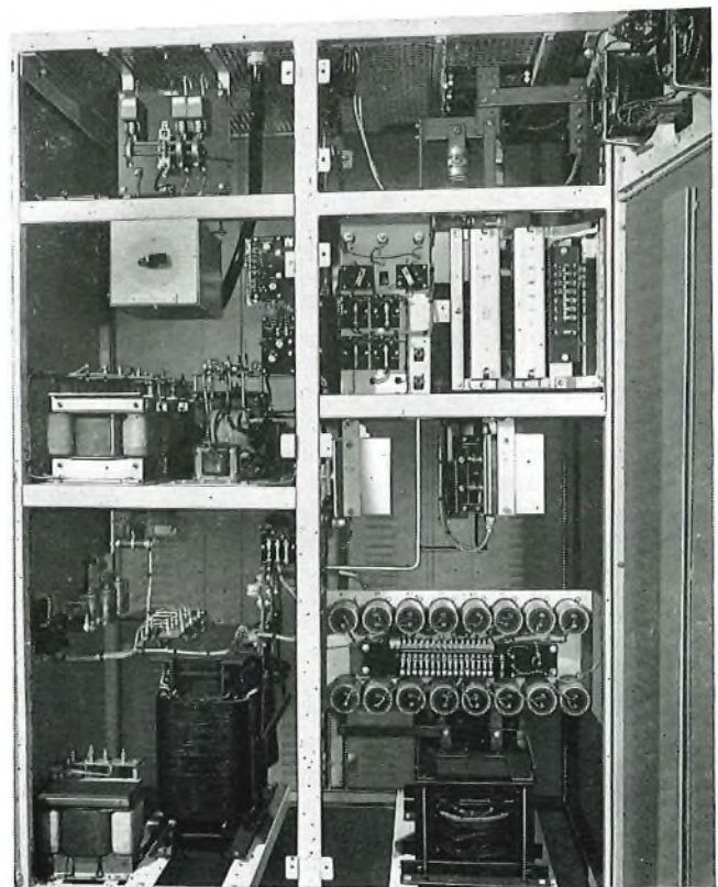
FIG. 15—Interior of a 200-amp load module
