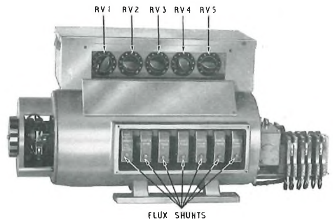
FIG. 1—DYNAMOTOR 43A
