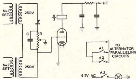
FIG. 6.—AUTOMATIC SYNCHRONISATION DETECTION UNIT.
