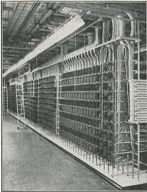
FIG. 5.—DISTRIBUTION FRAME.
