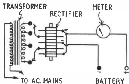
Fig. 1—Circuit
