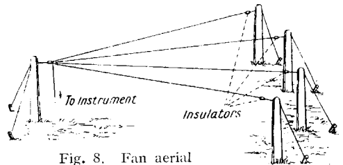
Fig. 8. Fan aerial
