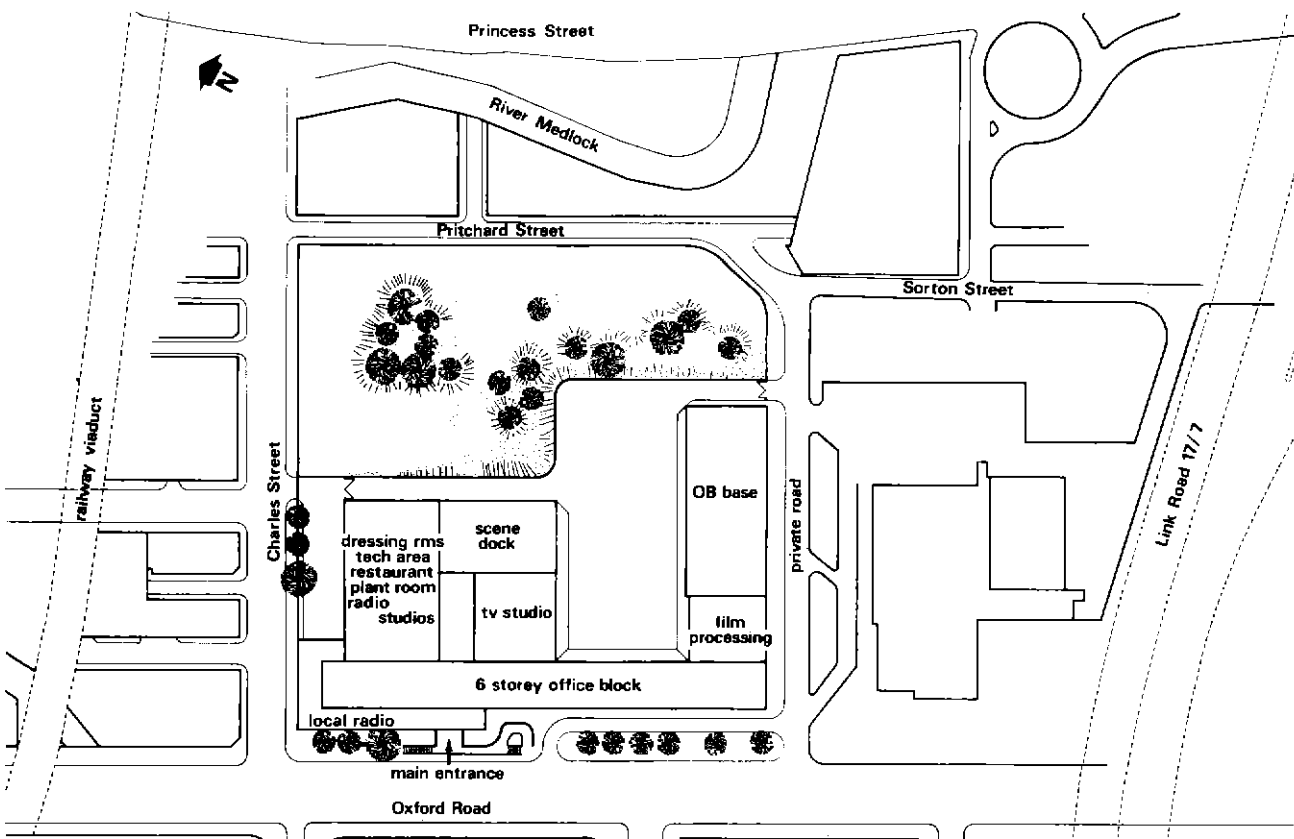
Fig. 2 The site layout
