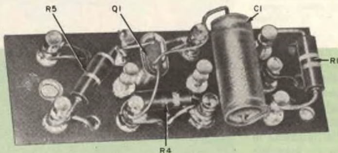
Tutti i componenti del dispositivo adattatore di impedenze sono montati su un pezzo di laminato plastico. La disposizione delle parti non è critica. L'unità può essere usata come un adattatore esterno o montata permanentemente in un apparato.
