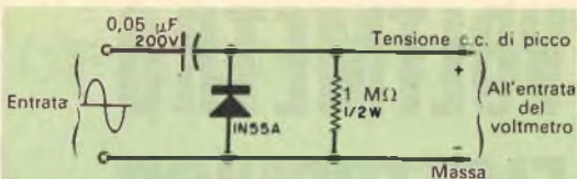
Sonda rivelatrice per la misura di basse tensioni di picco c.a. Per il filtraggio è sufficiente la capacità tra i fili della sonda stessa.
