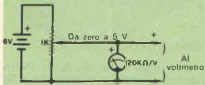
Fig. 3 - Circuito a tensione variabile usato per la taratura del voltmetro.
