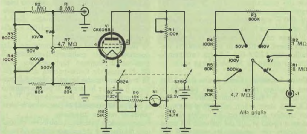
Fig. 1 - La caduta di tensione ai capi della resistenza catodica è proporzionale alla tensione da misurare. Quanto più positiva sarà la griglia tanto maggiore sarà la tensione ai capi della resistenza.
