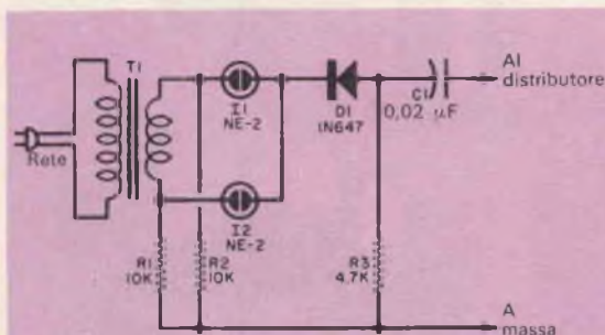
Fig. 2 - Gli impulsi provenienti dalla bobina di accensione dell'auto vengono scanditi dai 50 Hz della rete e fanno emettere dalle due lampadine al neon (I1 e I2) un segnale di calibratura.
