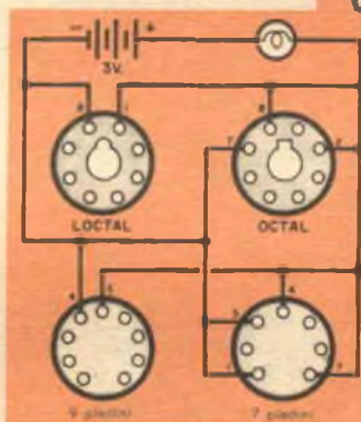
Fig. 1 - Un semplice provavacircuiti come quello rappresentato in figura è uno fra i tipi più semplici di provavalvole. Molto utile nella ricerca dei guasti, esso è munito di una lampada spia che si accende se i filamenti della valvola sotto prova sono in buone condizioni.
