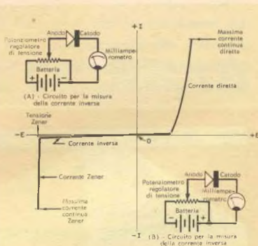
Fig. 1 - Le correnti dirette e inverse di un diodo Zener si possono misurare con semplici circuiti; la corrente inversa aumenta lentamente finché non si raggiunge il potenziale Zener.
