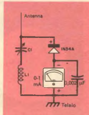
Fig. 2 - Sensibile misuratore di frequenza ad assorbimento che usa uno strumento da 1 mA fondo scala. Per misura di intensità del campo viene inserita una corta antenna.
