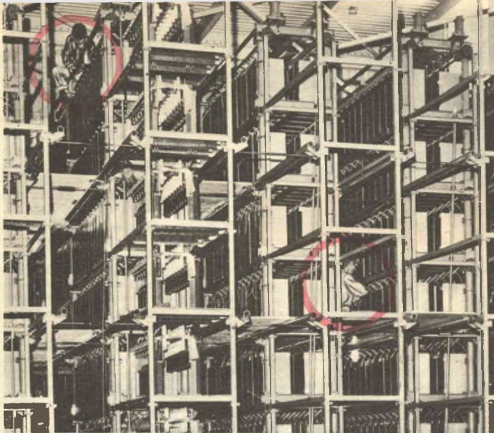
Il gigantesco banco di condensatori di Los Alamos (Nuovo Messico) produce una scarica di 40 milioni di ampere in 10 microsecondi. Gli operai, racchiusi nei cerchi, danno un'idea delle dimensioni complessive dell'apparecchio, del quale nella fotografia è rappresentata solo una terza parte.
