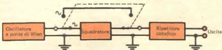
Fig. 1 - Schema a blocchi di generatore audio fornito di circuito squadratore che può essere incluso o escluso a piacere. Questo circuito squadratura l'onda sinusoidale data dall'oscillatore a ponte di Wien.
