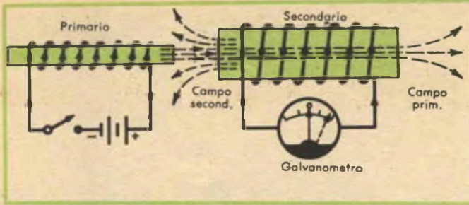
Fig. 5 - Il formarsi di un campo magnetico primario verso destra induce nel secondario una corrente elettrica che genera un campo verso sinistra. L'indice del galvanometro segna la direzione della corrente nell'avvolgimento secondario.
