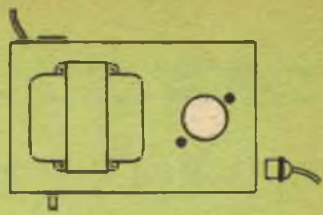
Fig. 2 - Telaio di alluminio su cui è montato l'alimentatore. Lungh. mm 230; larghez. mm 120; alt. mm 70.
