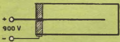
Fig. 5 - Applicazione della tensione all'elettrodo centrale del tubo Geiger.
