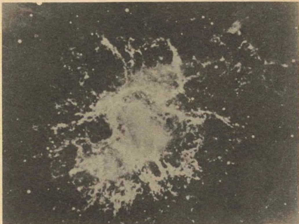
La « Crab Nebula » come appare agli obiettivi del telescopio di M. Palomar.
