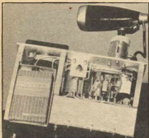
Veduta interna di un lato del fonometro. A sinistra è visibile la batteria alimentatrice del complesso.
