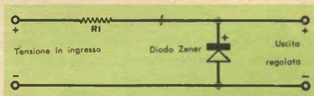
Fig. 2 - La scatola a sostituzione denominata Zeniac, offre la scelta tra undici diodi Zener da 1 W al silicio per tensioni comprese tra 3,6 e 30 V. Nello schema: come un diodo Zener viene usato quale regolatore di tensione.
