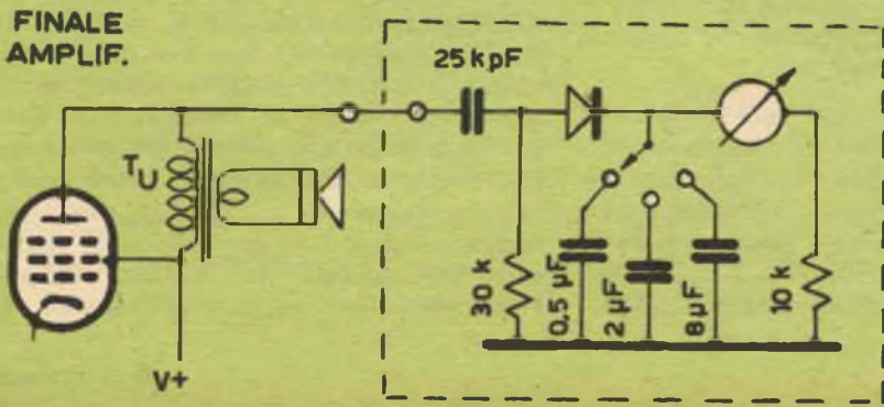
Fig. 6 - Nel caso si adoperasse l'amplificatore della radio, il terminale del condensatore deve essere inserito nella presa fono.
