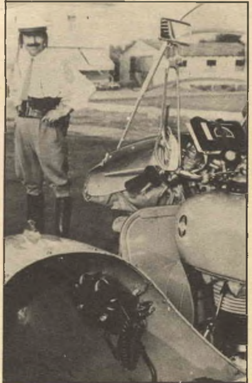
Il complesso ricetrasmittente montato sul sidecar della motocicletta.
