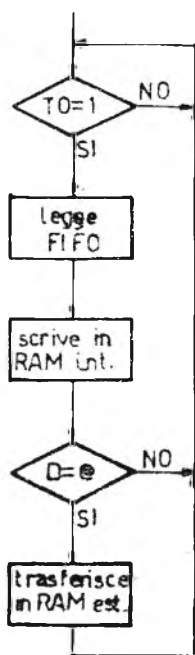
Figura 1 - Diagramma di flusso per lettura e memorizzazione dati.
