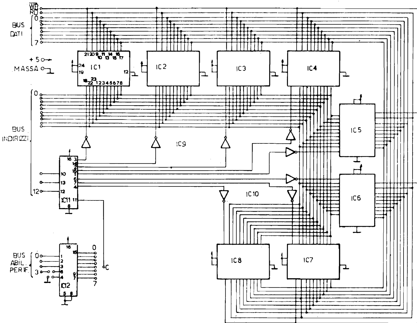
Figura 3 - Schema elettrico RAM 8K.
