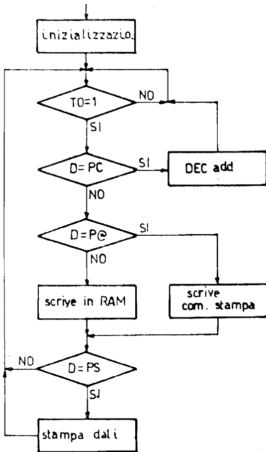
Figura 10 - Diagramma di flusso del programma di « stampa RAM ».
