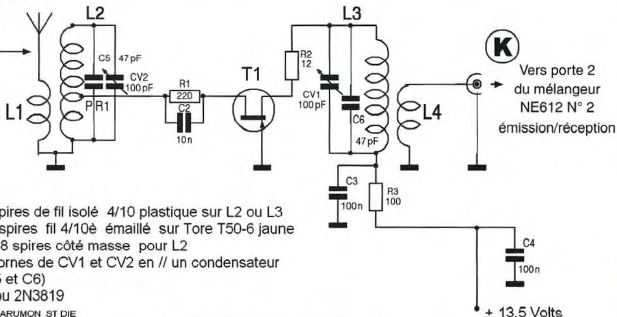
Figure 5 - Ampli HF réception : Schéma de principe.
