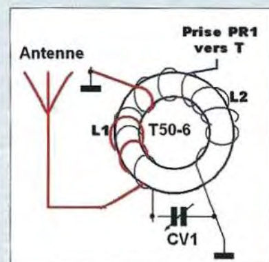
Figure 6 - Ampli HF réception : Disposition des enroulements sur L1 et L2.
