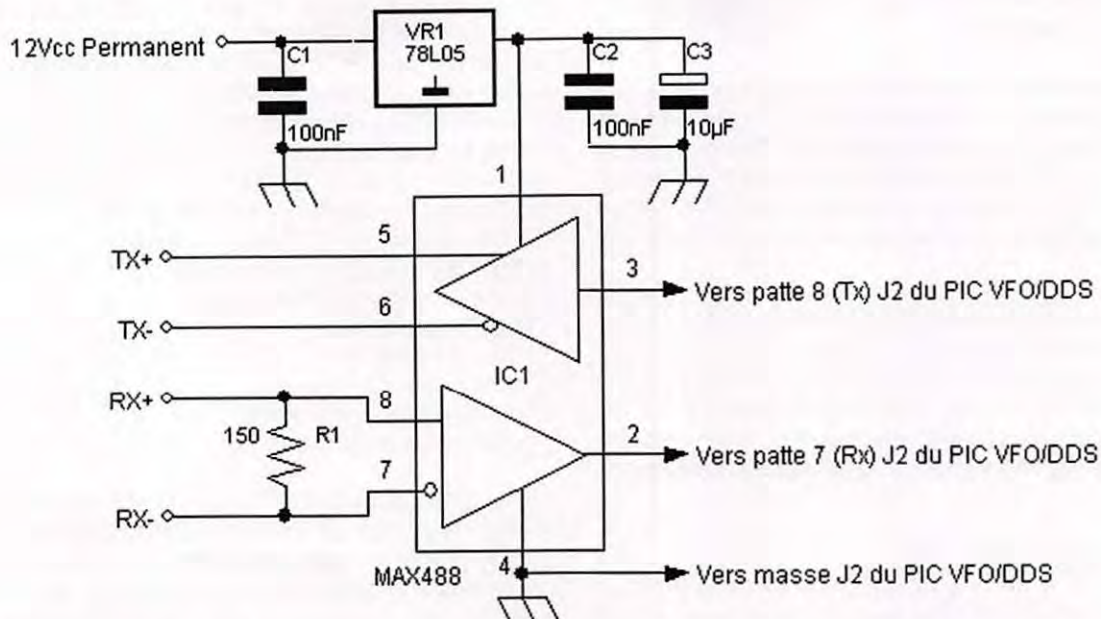
Schéma 6 - Le convertisseur RS422.
