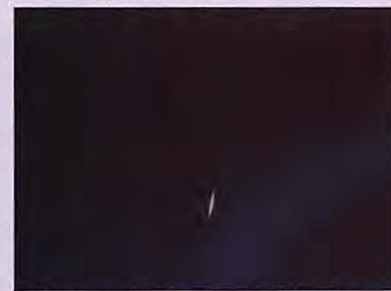
5 - Trace laissée dans le ciel lors d'un "flash" de satellite IRIDIUM.
