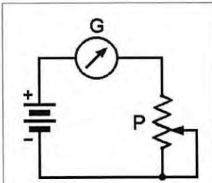
5 - Détermination de la résistance à mettre en série.
