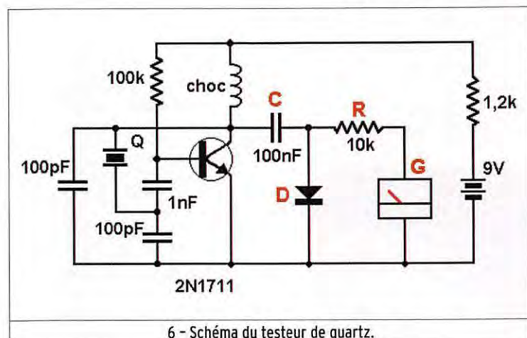
6 - Schéma du testeur de quartz.
