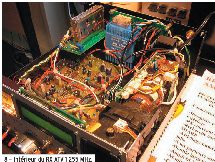
8 - Intérieur du RX ATV 1 255 MHz.
