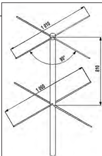
Fig. 8 - Réalisation pratique d'une antenne Turnstile.
