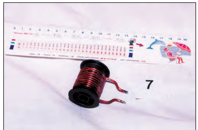
7 - Prototypé de bobinage pour filtre Chebyshev.
