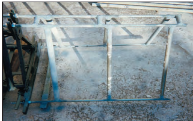
Photo n° 7 : Chaise en cours de construction et fixée sur le tronçon 1.
