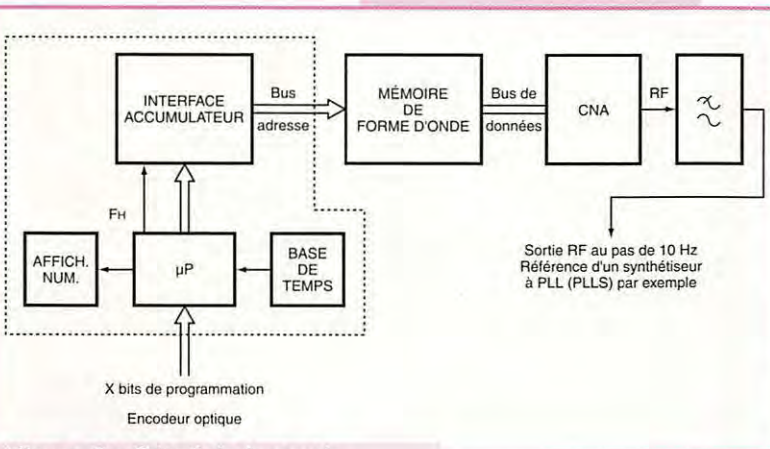
Figure 6 : Détail de la partie traitement.
