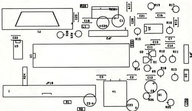
Implantation des composants. Ech. 1.
