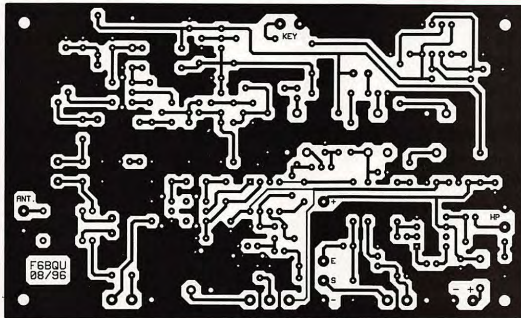
Circuit imprimé.
