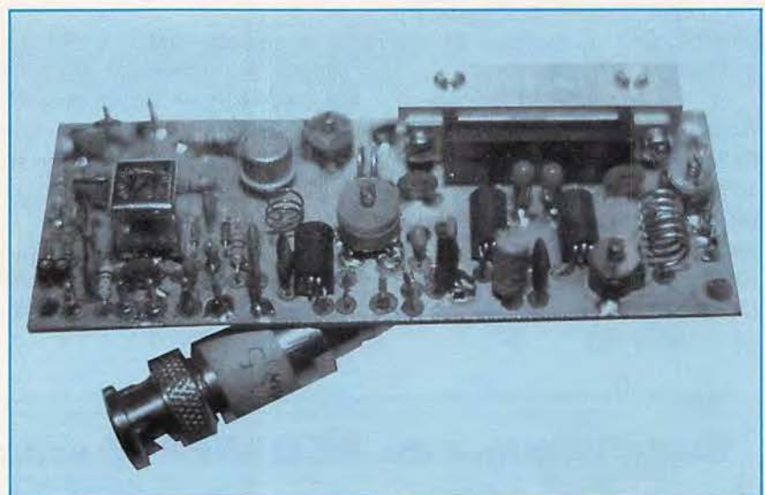
Vue générale de la nouvelle platine émission. Sur cette photo, la platine est en cours d'expérimentation.
