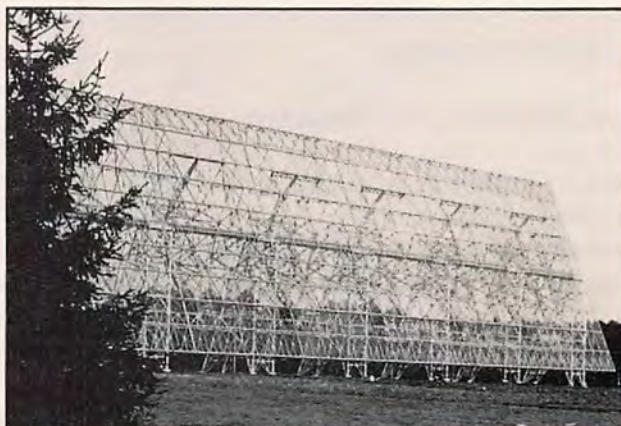
Le radiotélescope de Nançay : le miroir plan orientable.
