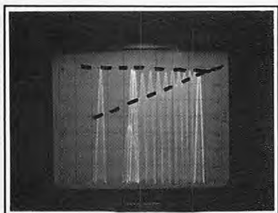
Photo E) Si la modulation n'est pas linéaire, les pics correspondant aux marches du signal ne sont pas équidistants, bien que les 10 marches du signal vidéo soient toutes de hauteur identique. De ce fait, les intersections entre les pics ne se font pas toutes à la même hauteur. C'est ce que nous avons souligné avec les deux lignes noires en pointillé. Pour réaliser cette photo, nous avons volontairement modifié le réglage des
