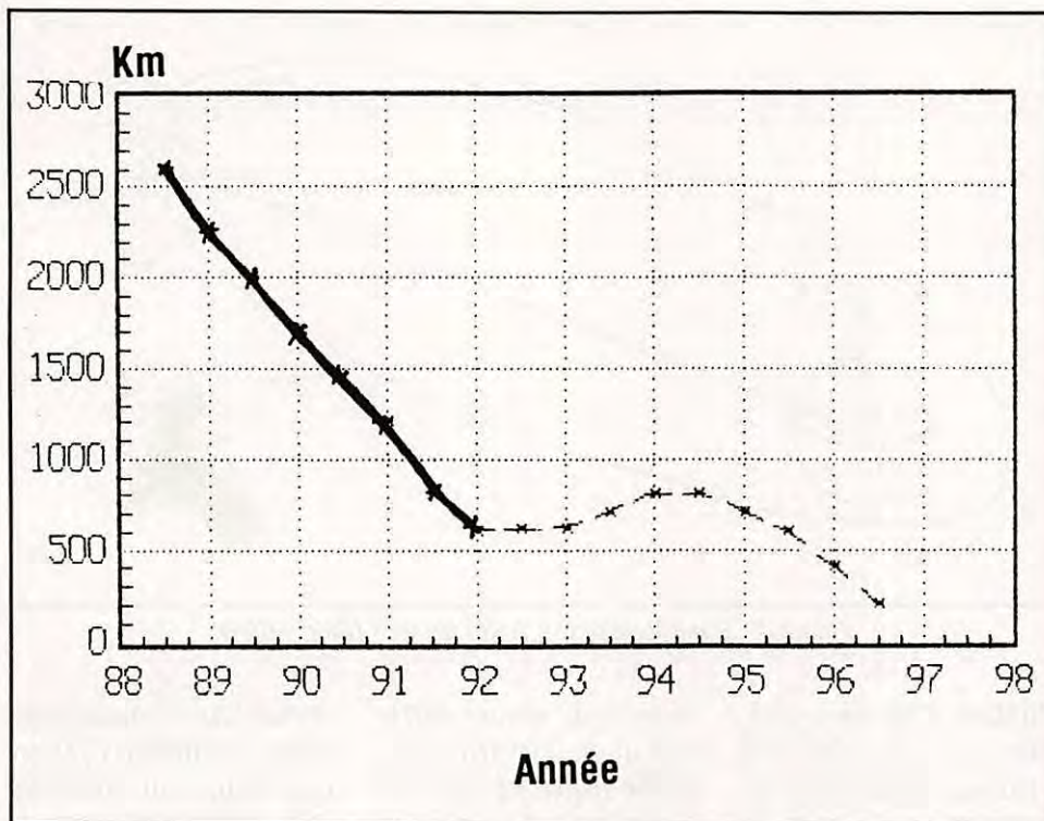
Figure 1 : OSCAR 13 : évolution passée et future de l'altitude du périhélie.
