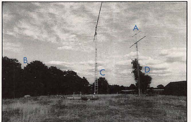
Le carré est tendu entre le pylône A et les arbres B, C et D.
