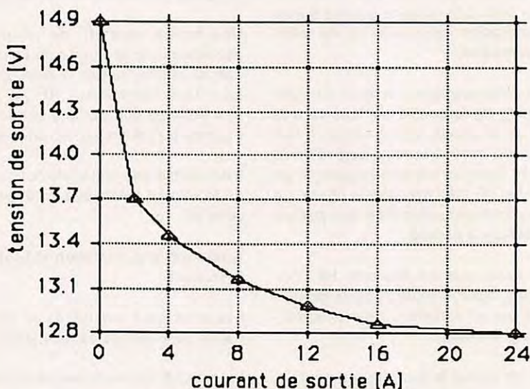
Figure 2 : Tension de sortie par rapport à la charge pour alimentation à stabilisation magnétique
