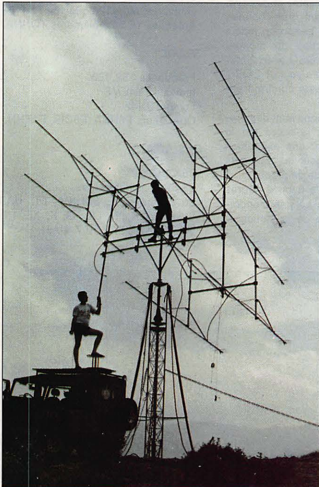
Photo 6 : Le montage des 4 groupes d'antennes après tests.
