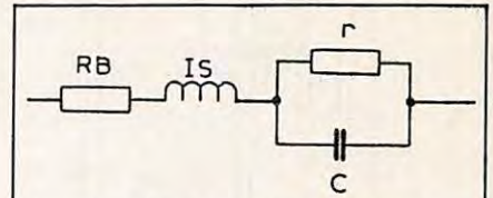
Figure 18 : Schéma équivalent de la diode tunnel
