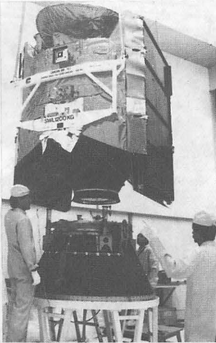
Intégration du satellite TĒLĒCOM 1-A dans la coiffe du lanceur ARIANE (Kourou).
