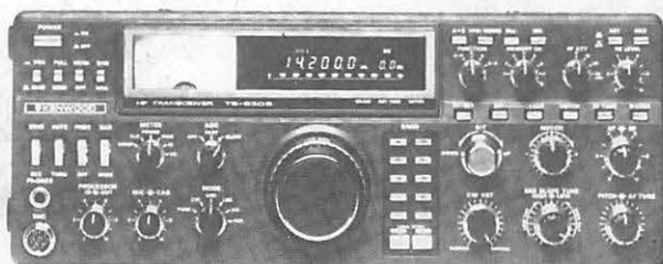
Emetteur-récepteur HF TS 930 SP* Emission bandes amateurs. Réception couverture générale tout transistor. AM/FSK/USB/LSB/CW. Alimentation secteur incorporée.
