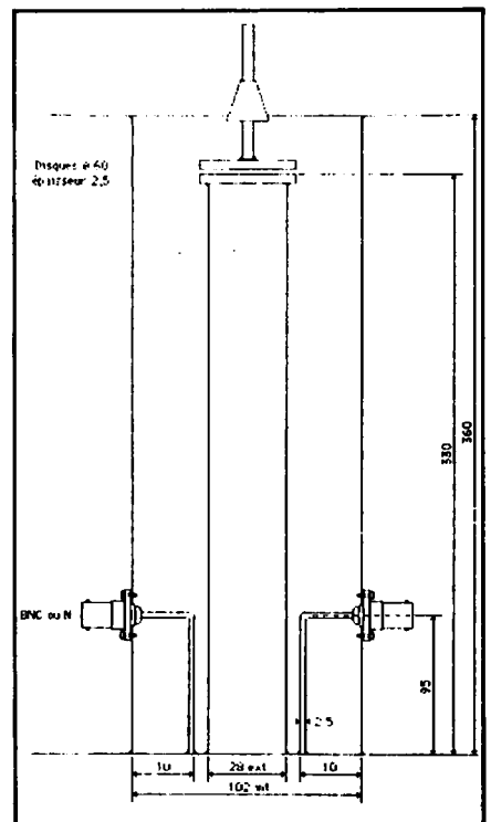
Figure 1 Cavité 144 — Z=50 Ω.
