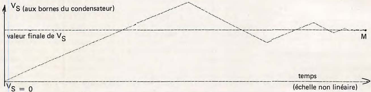
FIGURE 8 En éliminant les temps morts de la figure 7, on obtient une courbe plus exploitable.
