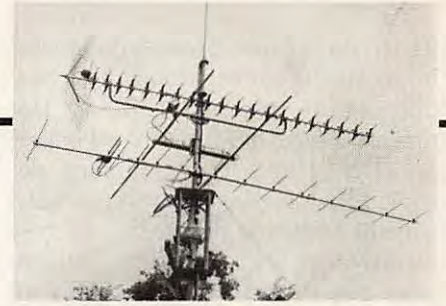
Les aériens de la station DX TV du Radio Club de Royan.
