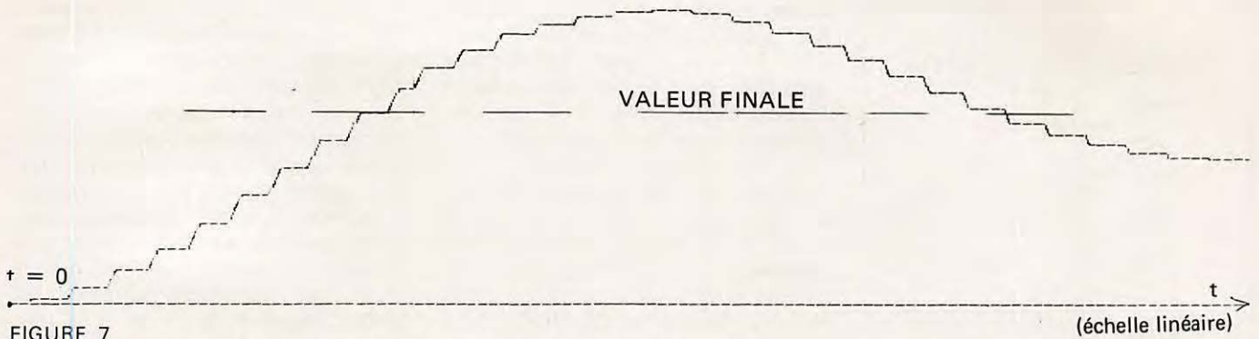
FIGURE 7 Evolution de la tension V_S (aux bornes du condensateur) en fonction du temps.
