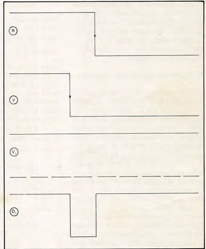
FIGURE 6 Vest en avance sur R. D_1 passe à 0 entre 2 fronts négatifs. Le système « estime » que la fréquence de Vest trop grande. Il va réagir de manière à diminuer celle-ci.
