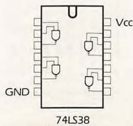
74LS38
