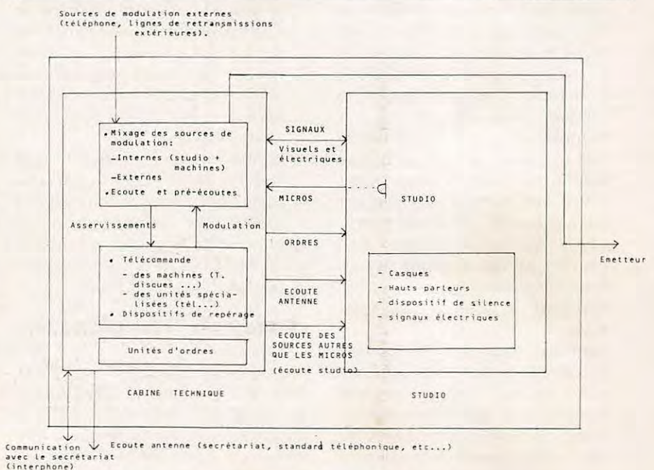
Figure 2 Système complet "studio-technique"
