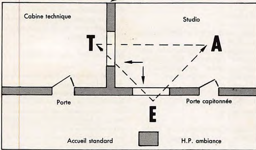
Figure 1 Dispositif possible du studio et de la cabine
