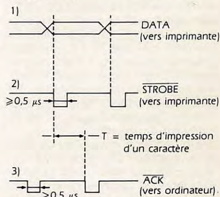
Figure 4 : Échange de données avec hand shaking
