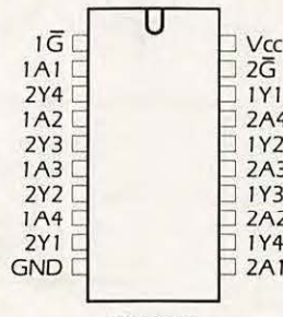
74LS244
