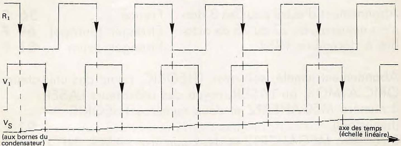
FIGURE 11 Simulation en temps réel du fonctionnement d'une boucle à CP séquentiel.
