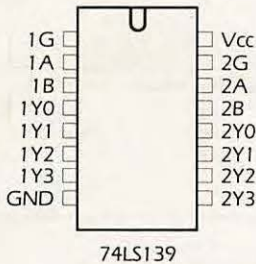
74LS139
