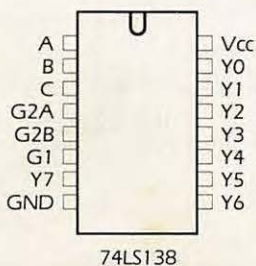
74LS138
