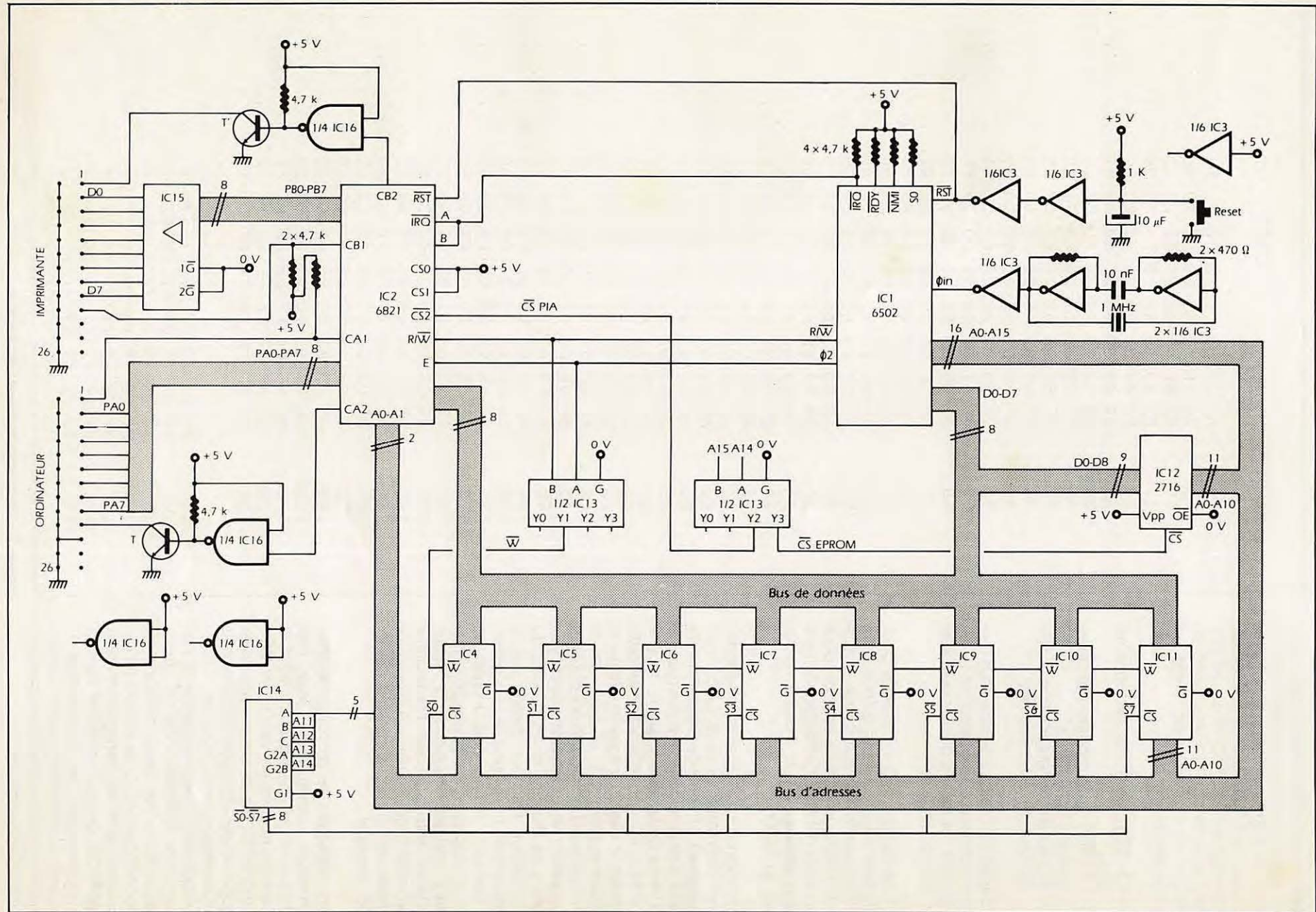
Figure 1 : Schéma électrique du buffer
