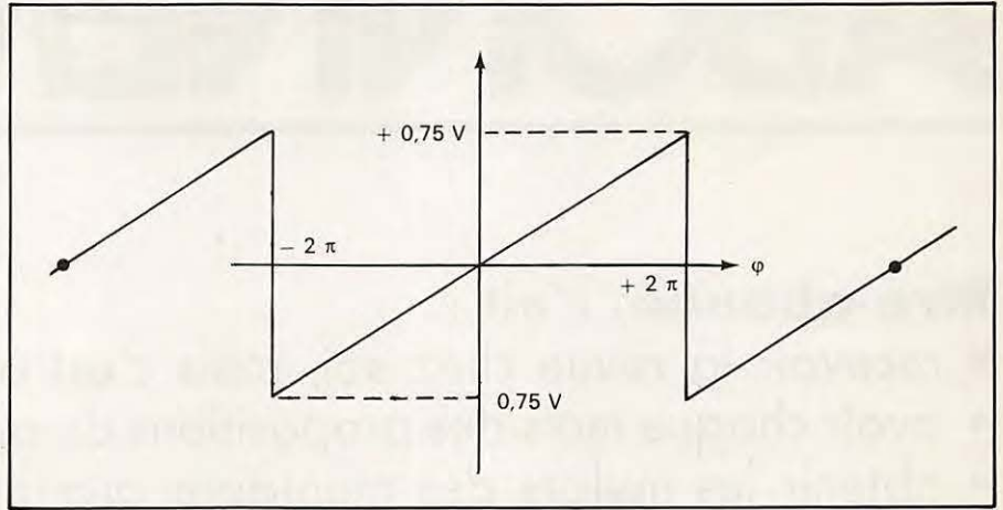
FIGURE 10 Variation de la tension moyenne de sortie.
