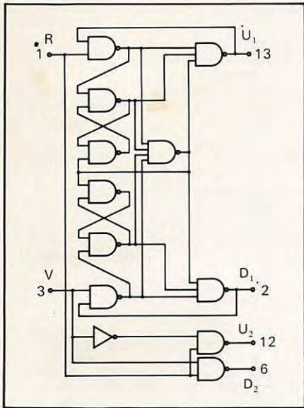
FIGURE 4b Les comparateurs de phases du MC 4344.
