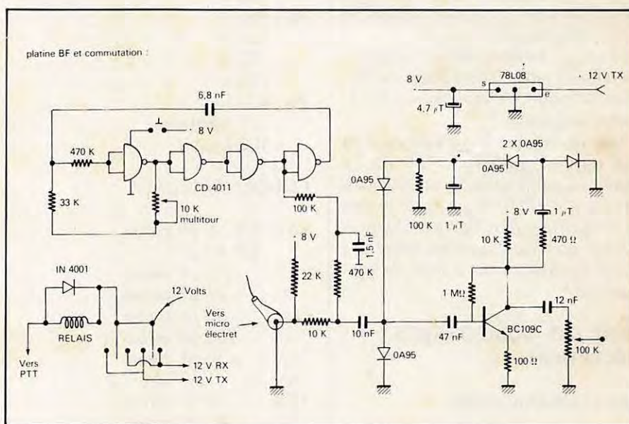
SCHEMA DE PRINCIPE
