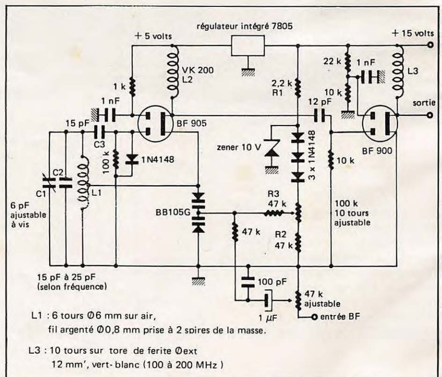
Schéma théorique de l'oscillateur
