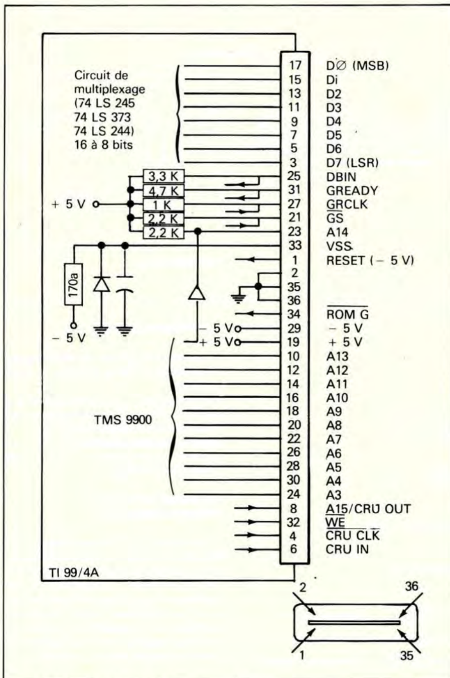
Figure 5 - CONNECTEUR GROM
