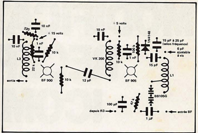
Implantation des composants Oscillateur
