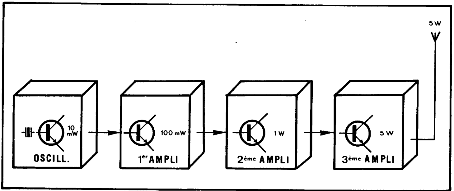
Figure 5 Trois étages amplificateurs HF confèrent à l'émetteur plus de puissance encore, et donc la possibilité d'envoyer le signal Haute Fréquence plus loin, de plus en plus loin ...
