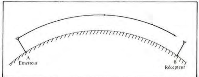
Fig. 1.3.2f. Avec un indice variant de 78.10^{-6}/\text{km} , l'onde pourrait suivre la courbure de la terre.
