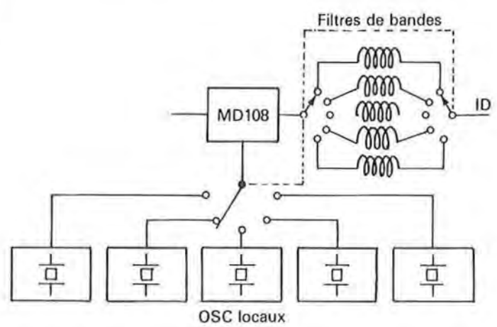
Modification pour l'obtention d'un TXVR 3, 5, 7, 14, 21, 28 MHz
