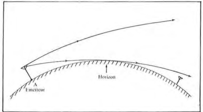
Fig. 1.3.2e. Pour une variation d'indice de réfraction normale ou inférieure à la normale, l'onde disparaît dans l'espace au-delà de l'horizon.
