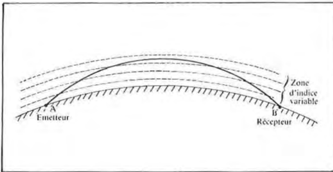
Fig. 1.3.2c. Si la variation d'indice est suffisante, l'onde peut être rabattue au sol.
