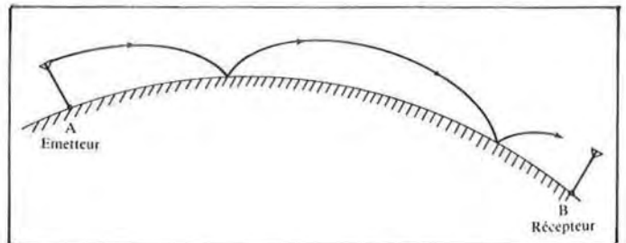
Fig. 1.3.2g. Pour une variation d'indice supérieure à 78.10^{-6}/\text{km} , l'onde ne peut s'échapper de l'atmosphère.
