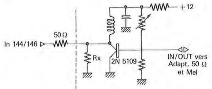
ATTENUATEUR DU TRANSVERTER
