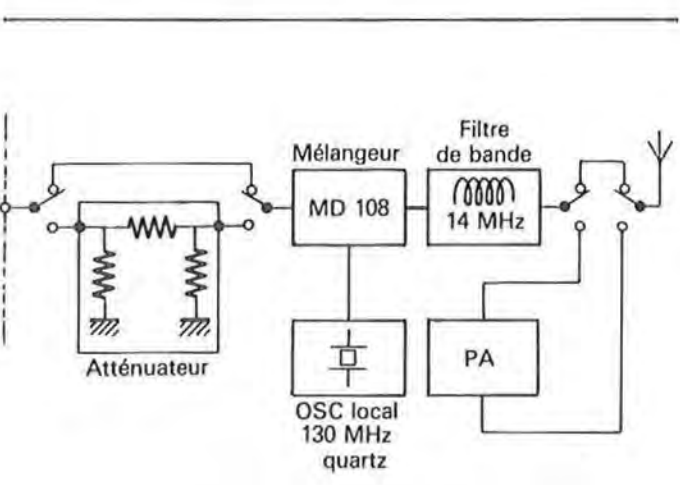
Schéma de base d'un transverter classique.
