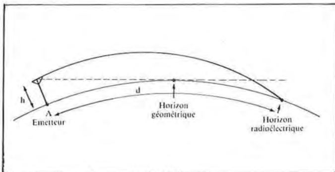
Fig. 1.3.2d. Si h est la hauteur de l'antenne au-dessus du niveau du sol, l'horizon radioélectrique d est donné par la formule d = 4,7\sqrt{h} avec d en km et h en m.
