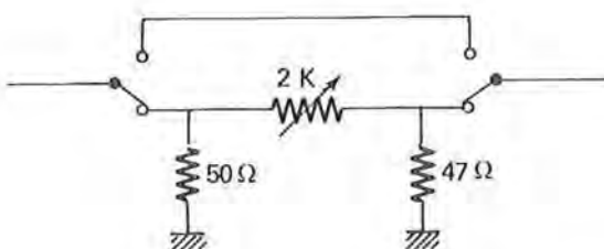
ATTENUATEUR
