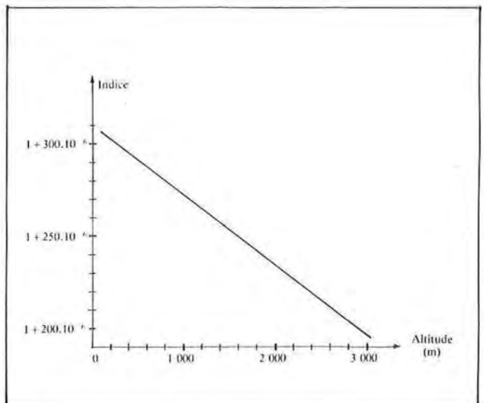
Fig. 1.3.2a. Variation de l'indice radioélectrique de l'atmosphère en fonction de l'altit.
