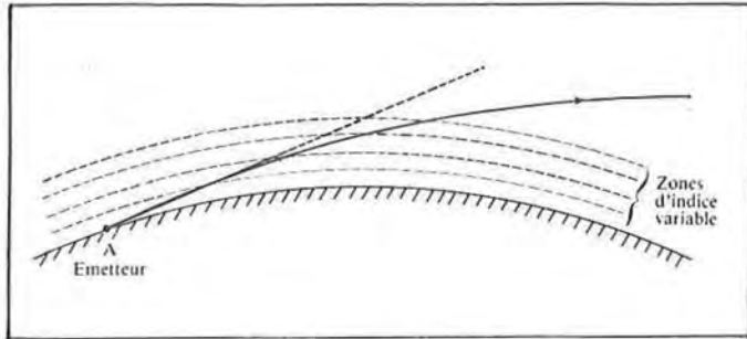
Fig. 1.3.2b. La variation d'indice de l'atmosphère en fonction de l'altitude courbe légèrement le trajet de l'onde.
