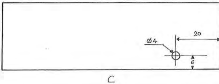
PLAN DE PERÇAGE DES BLINDAGÉS
