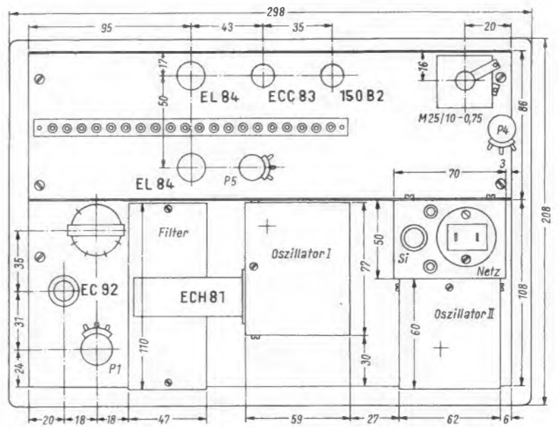
Rückansicht
