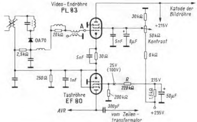
Der Widerstand R hatte seinen Wert erhöht, so daß sich der Arbeitspunkt der Tastpentode verschob. Infolge der zu geringen negativen Regelspannung wurde die Videoröhre übersteuert
