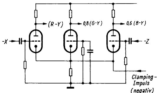
Bild 17. Matrix-Schaltung zur Gewinnung von (R - Y) , (B - Y) und (G - Y) aus X und Z
