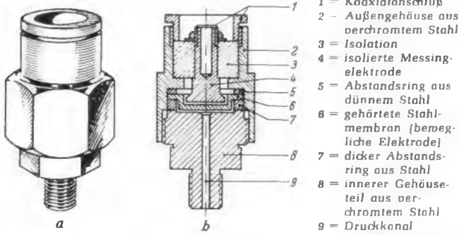
Bild 69. Äußere Form (a) eines kapazitiven Meßwertaufnehmers für große Drücke (Disa-Elektronik, Dänemark). Schnitt (b) durch den Hochdruckmeßwertaufnehmer
