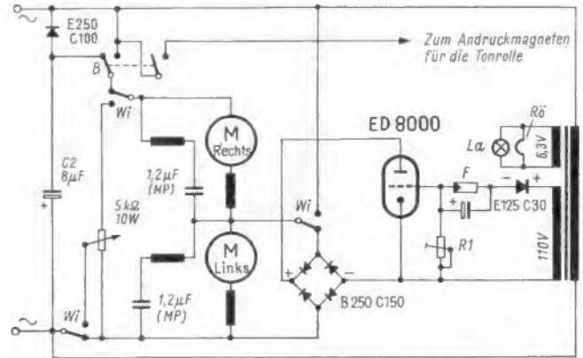
Links: Bild 7. Fühlhebelsmechanik mit Steuerung durch eine Foto-Elektronik
