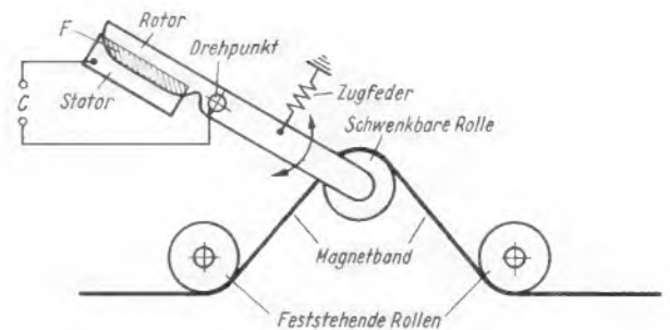
Bild 71. Aufbau einer Bandzugwaage mit einem kapazitiven Meßwert-aufnehmer (EMT, Franz KG, Lahr)
