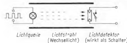
Bild 2. Prinzip eines Fotozerhackers
