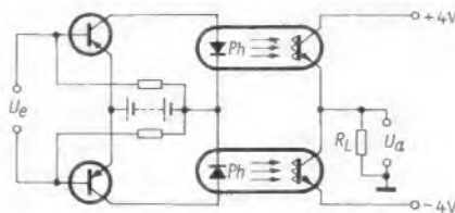
Bild 9. Symmetrischer Kleinsignal-Linearverstärker (Differenzverstärker) mit 230 dB Gleichtaktunterdrückung
