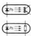
Bild 7. Von der FUNKSCHAU gewählte Symbole für optoelektronische Koppellemente. Im oberen Symbol dient ein Fototransistor als Detektor, im unteren eine Fotodiode
