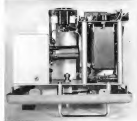
Bild 16. Seitenansicht des geöffneten Gerätes
