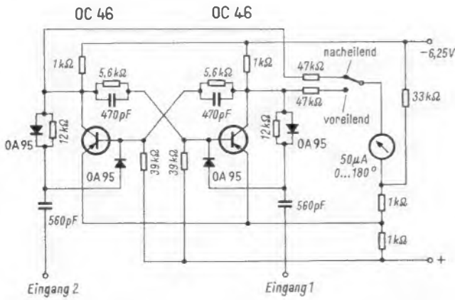
Bild 3. Flipflop-Stufe mit Anzeigeinstrument. Diese Stufe ist in England als kompletter vergossener Baustein, Typ B 8 92000, von Mullard zu beziehen (ohne die Anschaltung)
