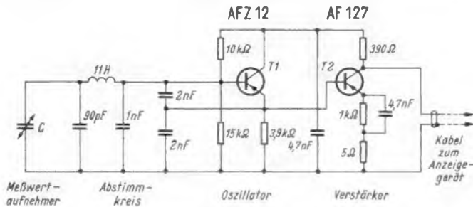
Bild 70. Schaltung des Elektroniketeiles für den Meßwertaufnehmer von Bild 69
