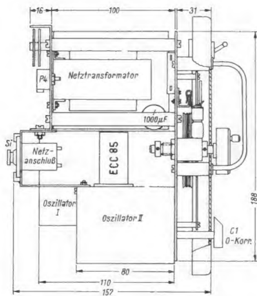
Rechte Seitenansicht
