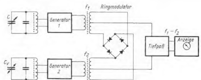
Bild 72. Prinzipschaltung der elektronischen Bandzugwaage für Tonbandgeräte. Der kapazitive Meßwertaufnehmer C liegt im Schwingkreis des einen Transistorgenerators, der des zweiten ist mit Hilfe des Kondensators C_v einzustellen, um eine günstige Differenzfrequenz für die Anzeige zu erhalten
