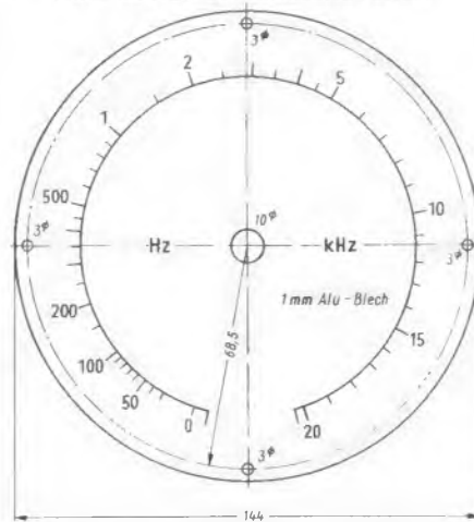
Bild 14. Die Skala mit der im Mustergerät geeichten Frequenzteilung
