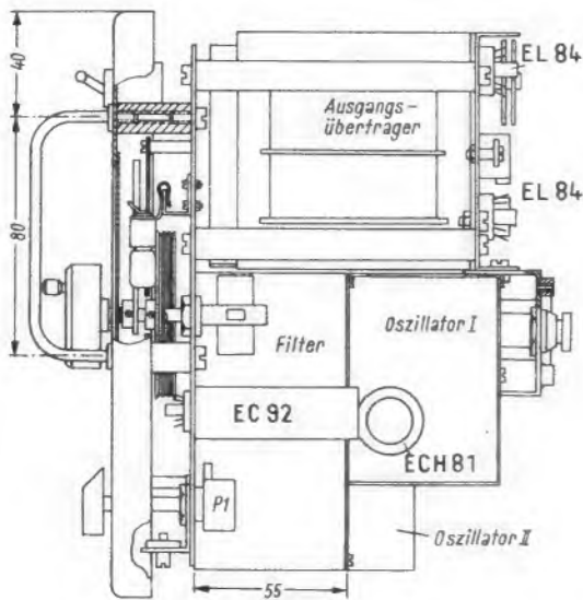
Linke Seitenansicht
