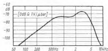
Bild 2. Der Frequenzgang ist bewußt für gute Spracherständlichkeit ausgelegt
