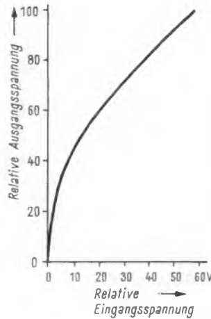
Bild 23. Kennlinie des \gamma -Korrektors, für \gamma = 2,2 (nach [1])
