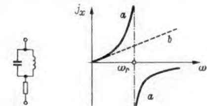
Bild 3. Ersatzschaltbild einer realen Spule und Verlauf des Blindwiderstandes; a = reale Spule, b = ideale Induktivität
