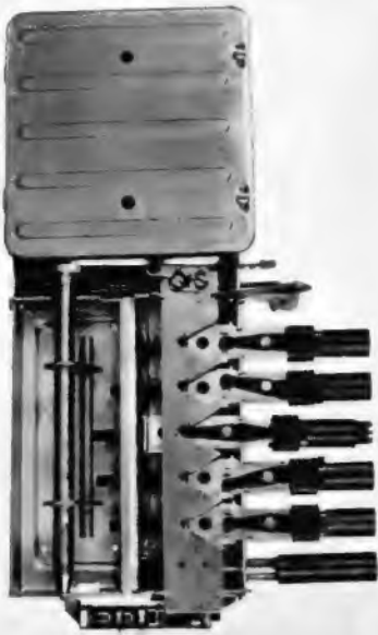
Bild 2. Einblock-Tuner von Blaupunkt mit Tastensatz. Die Einstellung auf den Bereich wird durch Drehen der Tastenhülsen vorgenommen und die Abstimmung auf den Sender mit Hilfe der Spindeln in den Tastenhülsen
