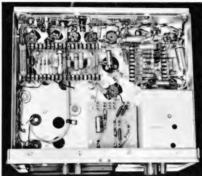
Bild 5. Unteransicht des Chassis des Verstärker-Voltmeters TF 2600
