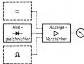
Bild 1a. Prinzip des sogenannten Universalvoltmeters (Diodenvoltmeter)
