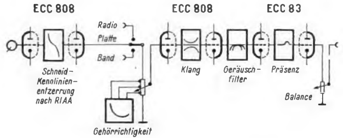
Bild 6. Blockschaltung des Steuerverstärkers
