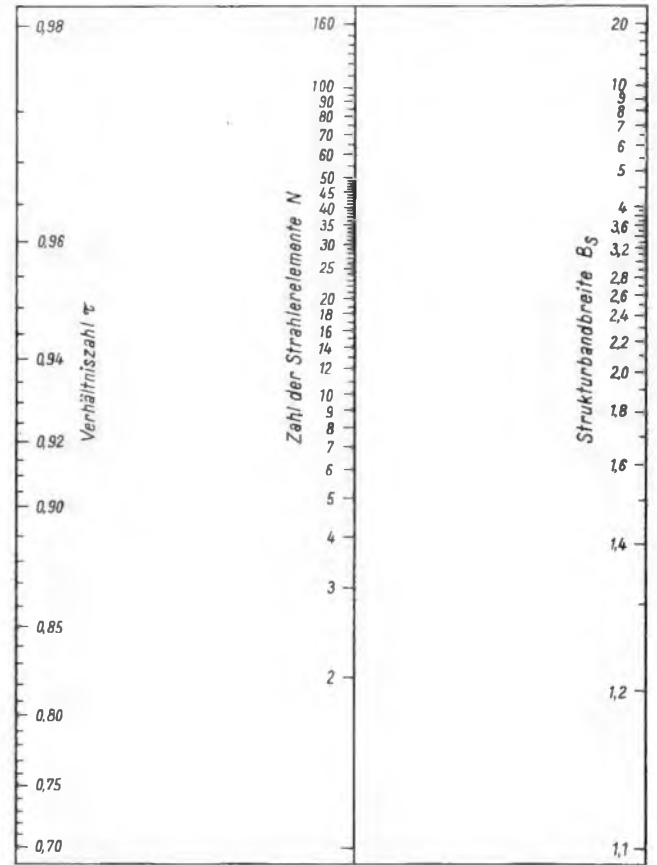
Bild 14. Nomogramm für die Beziehung: N = 1 + \frac{\log B_S}{\log \frac{1}{\tau}}
