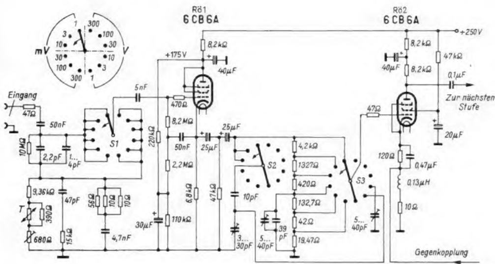
Bild 4. Ausführliche Schaltung des Eingangsteiles
