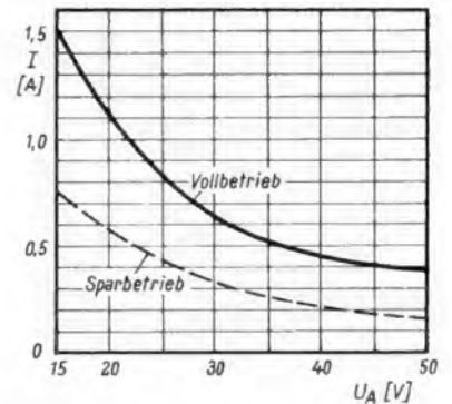
Bild 3. Die Kurven geben an, welcher Strom maximal entnommen werden kann, ohne daß die Stabilisierung aussetzt
