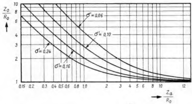
Bild 17. Relativer Widerstand der Speiseleitung \frac{Z_0}{R_0} in Abhängigkeit vom relativen Dipolwiderstand \frac{Z_a}{R_0} für mehrere Werte von \sigma'
