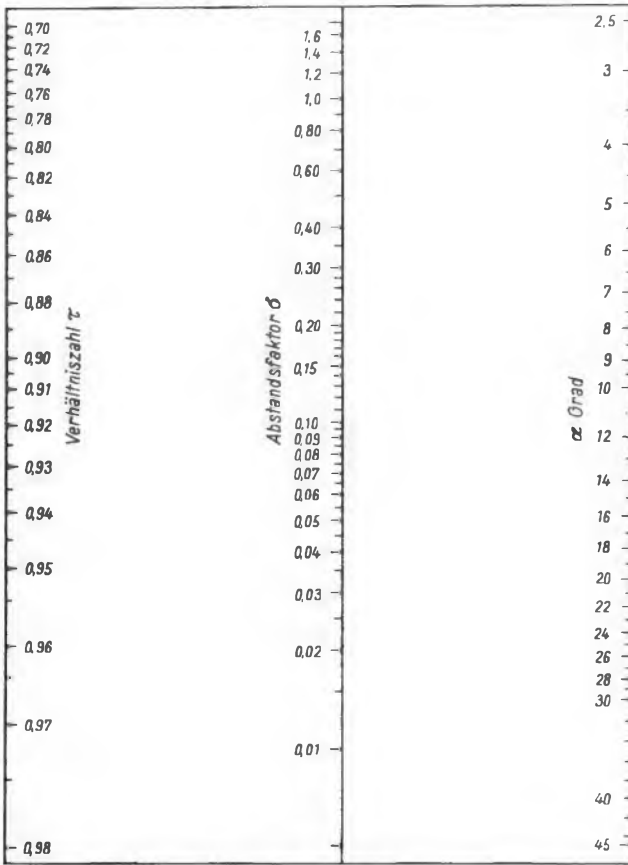
Bild 12. Nomogramm für die Beziehung: \sigma = \frac{1}{4} (1 - \tau) \cot \alpha
