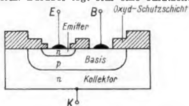
Schnittzeichnung eines Planarsystems
