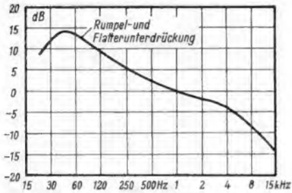
Bild 8. Frequenzkurve des Schneidkennlinienentzerrers, gemessen am Gitter 1 der zweiten Röhre. Lautstärke voll aufgedreht U_e am Phono-Eingang = 1,7 mV const., Gehörlichkeit ausgeschaltet
