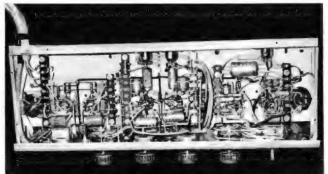
Bild 4. Blick in die Verdrahtung des Steuerverstärkers
