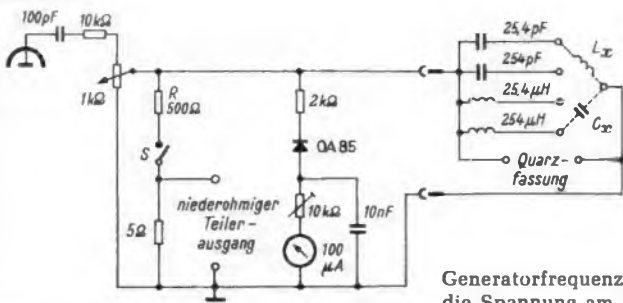
Bild 2. Ausgangsschaltung des vom Verfasser verwendeten Prüfsenders. Der Schalter S zum Auftrennen des niederohmigen Spannungsteilers und der Instrumentenzweig wurden zusätzlich eingebaut. Meßkondensatoren und Meßspulen werden außen angesteckt
