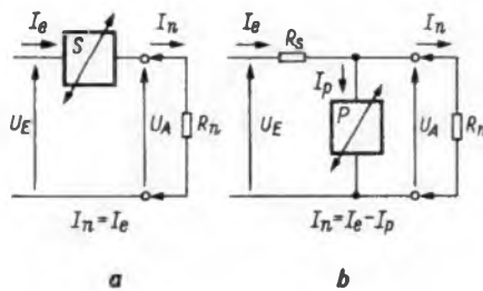
Bild 2. Die Prinzipbilder veranschaulichen den Unterschied von Serienregelung (a) und Parallelregelung (b) eines stabilisierten Netzgerätes
