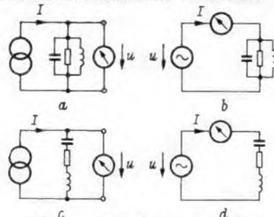
Bild 1. Vier Möglichkeiten zur Resonanzbestimmung
