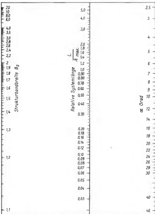
Bild 13. Nomogramm für die Beziehung: \frac{L}{\lambda_{max}} = \frac{1}{4} \left(1 - \frac{1}{B_S}\right) \cot \alpha
