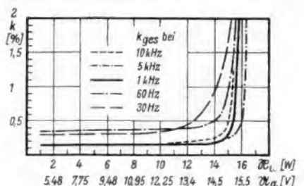
Bild 11. Klirrfaktor als Funktion der Ausgangsleistung; Abschlußwiderstand 15 \Omega , reell; U_e = 9,7 mV const.; Bässe und Höhen in Mittelstellung
