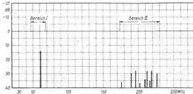
Bild 5. Korrigiertes Störpektrum von Bild 4
