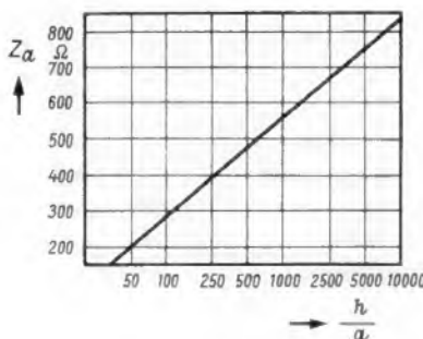
Bild 16. Mittlerer Wellenwiderstand eines Dipolstabes
