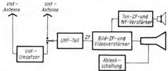
Bild 1. Blockschaltung eines Fernsehempfängers mit VHF-Umsetzer
