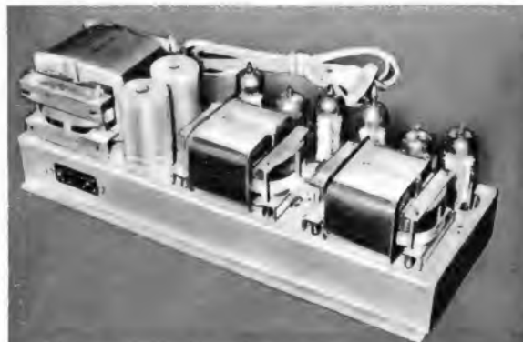
Links: Bild 2. Der Endverstärker. Gut zu erkennen sind die Ausgangsübertrager mit Schnittbandkernen und die versenkt angeordneten Röhren EL 84
