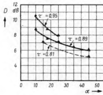
Bild 15. Abhängigkeit der Richtschärfe D von \alpha und \tau
