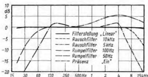
Bild 10. Filterfrequenzgangkurven, gemessen ab Eingang „Radio“. Lautstärke voll aufgedreht
