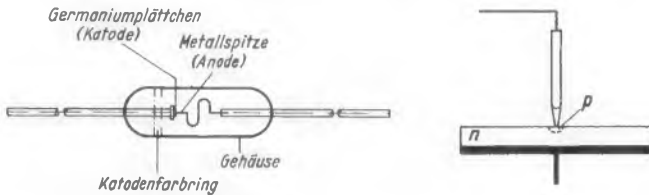
Bild 11.1. Schnitt durch eine Punktkontakt-Diode
