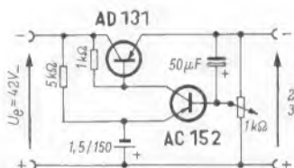
Bild 3. Geregelter Netzteil für Ausgangsspannungen zwischen 2 und 20 V bei maximal 300 mA Ausgangsstrom
