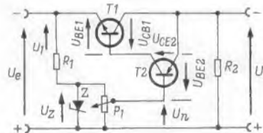
Bild 5. Grundsätzliche Schaltung eines geregelten Transistor-Netzteils mit großem Ausgangsspannungsbereich und hoher Regelgenauigkeit
