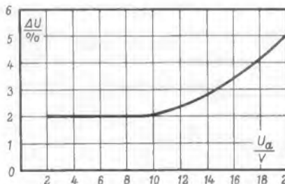
Bild 4. Belastungskennlinie des Netzteils nach Bild 3
