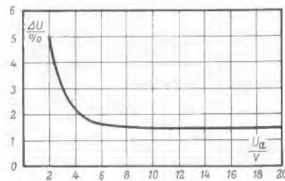
Bild 7. Belastungskennlinie des Netzteils nach Bild 6
