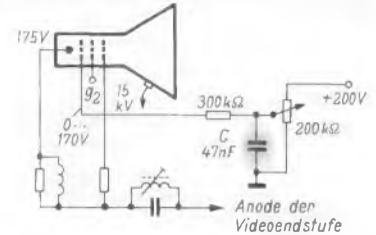
Bild 1. Die Bildröhre war dunkelgesteuert, da die positive Spannung am Wehneltzylinder fehlte. Ursache war ein Durchschlag des Kondensators C
