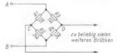
Bild 2. Darstellung der ersten vier Widerstände des Netzwerks als abgeglichene Brücke
