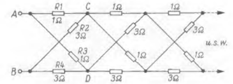
Bild 1. Welchen Widerstandswert weist dieses Netzwerk zwischen den Punkten A und B auf?
