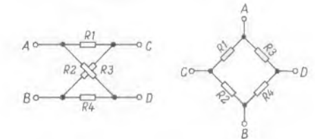
Bild 3. Vergleich zwischen einer Brücke als X-Schaltung und der gebräuchlichen Wiedergabe
