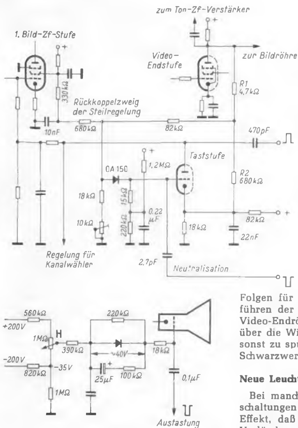
Bild 5. Neue Leuchtfleck-Unterdrückungsschaltung
