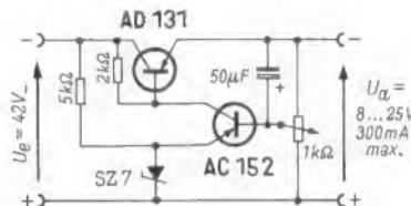
Bild 1. Geregelter Transistor-Netzteil für Ausgangsspannungen zwischen 8 und 25 V bei maximal 300 mA Ausgangsstrom
