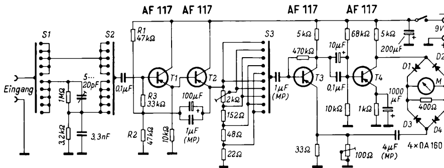
Schaltung eines Transistor-Breitband-Millivoltmeters
