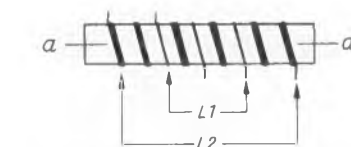
Bild 15. Zum Abgleich des Vorkreisstreifens werden die äußeren Windungen a verbogen
