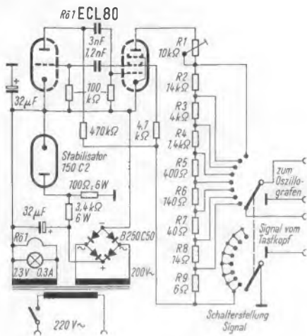
Bild 20. Schaltbild eines leicht zu bauenden Eichgenerators für Elektronenstrahl-Oszillografen
