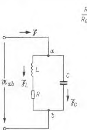
Bild 1. Parallelresonanzkreis
