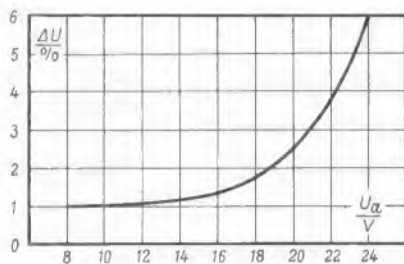
Bild 2. Belastungskennlinie des Netzteils nach Bild 1
