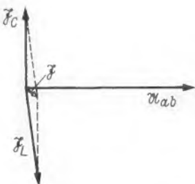
Bild 2. Vektordiagramm für den Parallelresonanzkreis
