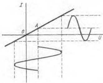
Bild 11.6. Gleicher Vorgang wie in 11.5, aber Arbeitspunkt durch eine „Vorspannung“ von 0 nach A verschoben
