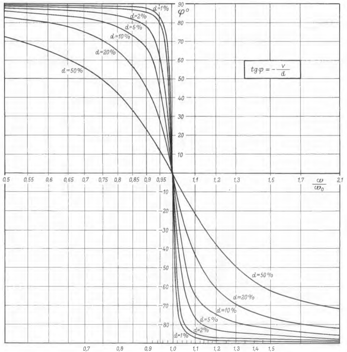
Bild 5. Normierter Phasenverlauf
