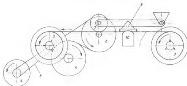
Bild 2. Das Antriebsprinzip des Tonbandteils. 1 = Tonband, 2 und 3 = Wickelteller, 4 = Motor, 5 und 6 = gegensinnig laufende Schwunzscheiben, 7 = Andruckrolle, 8 = Flachriemen, 9 = Bandführung, 10 = Tonkopf
