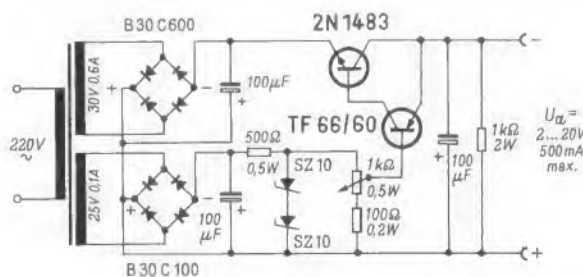
Bild 5. Grundsätzliche Schaltung eines geregelten Transistor-Netzteils mit großem Ausgangsspannungsbereich und hoher Regelgenauigkeit
