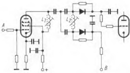
Bild 17. Automatik-Baustein mit Abgleichpunkten. Das Triodensystem der Verbundröhre dient als Gleichspannungsverstärker
