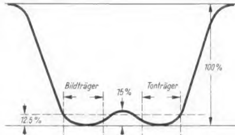
Bild 13. Hf-Normkurve. Die Toleranzgrenzen für die Welligkeit sollen nicht überschritten werden
