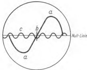
Bild 12. Abgleichen des Diskriminators: Die Kurve a wird beim Abgleich des Ton-Diskriminators auf größte Symmetrie eingestellt. Dann wird die quarzkontrollierte Marke b exakt auf den Nulldurchgang gebracht. Anschließend wird auf 800-Hz-AM-Modulation umgeschaltet und mit dem Trimmwiderstand des Diskriminators die Schwebung c auf Minimum abgeglichen
