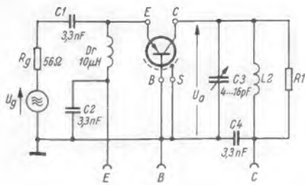
Bild 4. Meßanordnung zur Bestimmung der VHF-Leistungserstärkung des Transistors GF 132.
