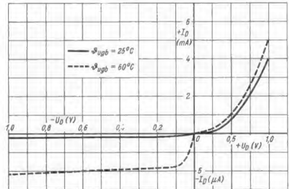
Bild 11.9. Kennlinien einer modernen Punktkontakt-Diode (Valvo)
