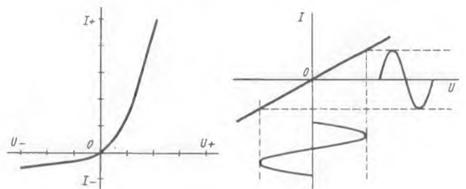
Bild 11.4. Beispiel einer nicht-linearen Kennlinie
