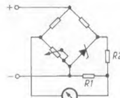
Schaltung einer temperaturkompensierten Zenerbrücke zur Überwachung der angelegten Spannung
