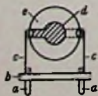
Links: Bild 4. Alterer Quarzaufbau: Quarzscheibe (Dickens-Scherschwingler) zwischen zwei Elektroden mit Luftspalt
