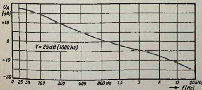
Bild 3. Frequenzcharakteristik der Entzerrerstufe für dyn. Tonabnehmer mit EF 86 in Pentodenschaltung im Verstärker NG 5601
