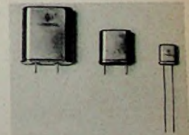
Bild 15. Drei moderne Siemens-Quarze in Metallhalter, rechts eine Subminiaturausführung mit Lötdrähten
