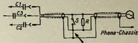
Bild 3. Im Plattenspieler ist u. U. die gestrichelt gezeichnete Verbindung aufzutrennen
