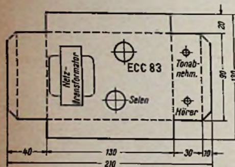
Bild 5. Maßzeichnung des Geräte-Chassis
