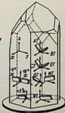
Bild 2. Wie die verschiedenen Quarzschnitte im Quarzkristall liegen
