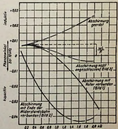
Bild 4. Phasenwinkel zwischen Spannung und Strom bei Schaltung nach den Bildern 1 bis 3
