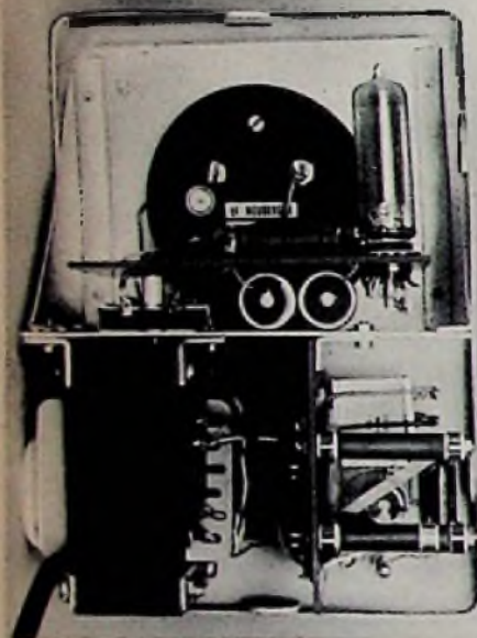
Bild 3. Ansicht des Chassis von der Rückseite aus gesehen
