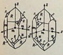
Bild 1. Die ideale Quarzgeometrie, a) Rechtsquarz, b) Linksquarz
