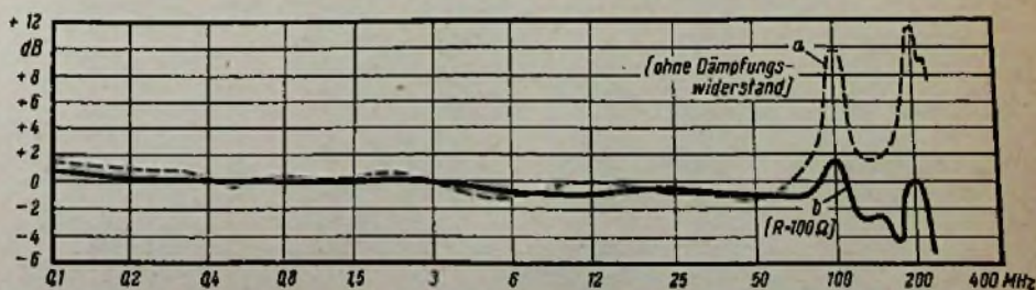
Bild 9. Durchlaßkurven im HF-Gebiet
