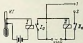
Bild 2. Schaltanordnung zur Temperaturregulation. KT = Kontaktthermometer, das möglichst in unmittelbarer Nähe der Transistoren zu montieren ist. I = Feinrelais, in Arbeitsstellung gezeichnet, II = Schaltschütz. 1, 2 = Anschlüsse für den Wärmestrahler
