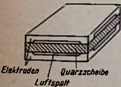
Links: Bild 4. Alterer Quarzaufbau: Quarzscheibe (Dickens-Scherschwingler) zwischen zwei Elektroden mit Luftspalt
