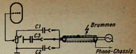
Bild 2. Bei einer zweiadrigen abgeschirmten Schnur kommen Mantelströme nicht in den NF-Weg
