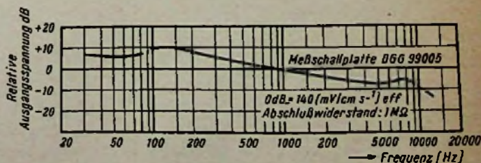
Bild 2. Frequenzkurve der Keramik-Tonabnehmersysteme Elac BST 1 und BST 2 bei Mikro rillenabstimmung, bezogen auf konstante Auslenkgeschwindigkeit
