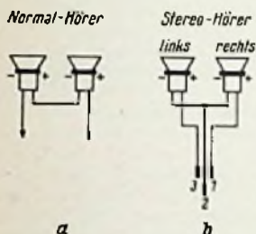
Bild 1. Schaltungen eines Stereo- und eines Normal-Kopfhörers
