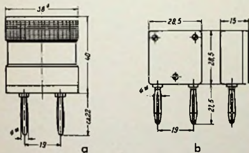
Bild 10. Maßskizzen von Preßstoffhaltern (Dr. Steeg & Reuter). a) ältere runde Form, b) neuere flache Form
