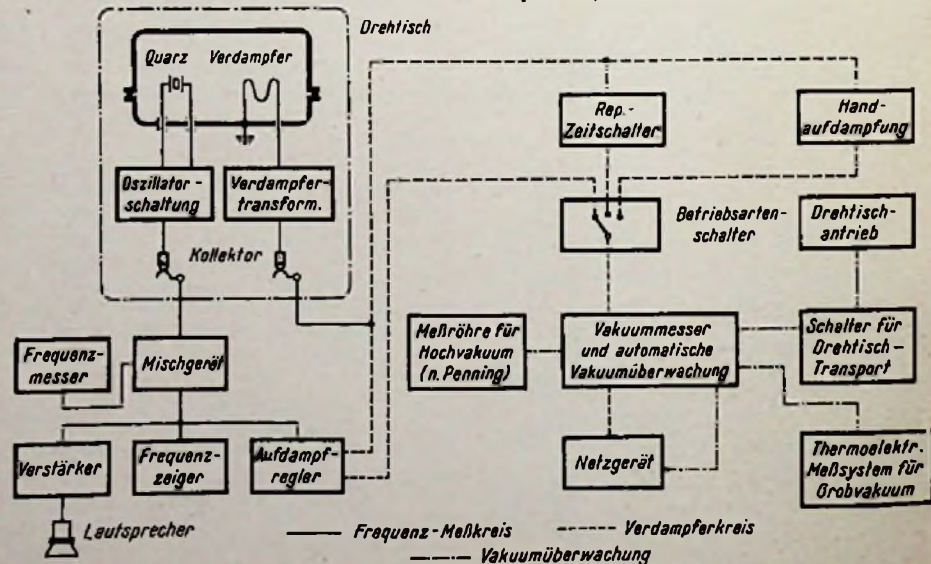
Bild 7. Blockschaltdiagramm der von Telefunken entwickelten Quarz-Aufdampfanlage
