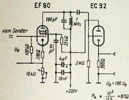
Bild 7. Hilfsschaltung zum Erzeugen genügend großer Eichspannungen
