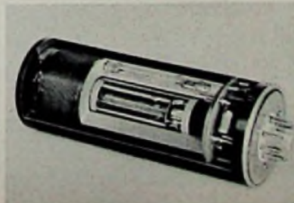
Bild 13. Diese Miniatur- und Subminiaturquarze gehören in die in Bild 12 gezeichneten Kappen
