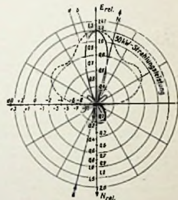
Bild 7. Strahlungsdiagramm der UKW-Rundfunkantenne in Band II; a) horizontal, b) vertikal
