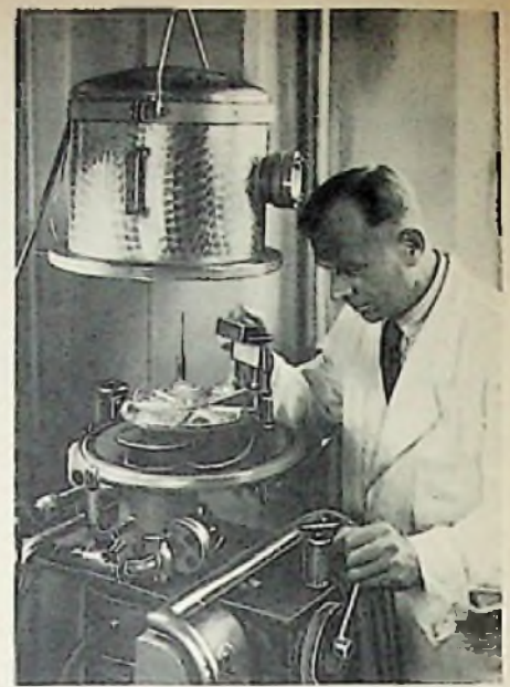
Bild 6. Aus der Schwingquarzfertigung bei Siemens: Aufbringen der Schichtelektroden im Vakuum-Pumpstand mit Kolodenzersäubung
