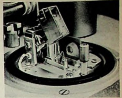
Bild 9. Innenansicht eines der Rezipienten; Haube für Frequenzaufdampfung (Feinaufdampfung) offen
