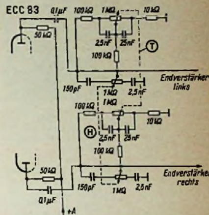
Bild 8. Doppelseitig wirkendes Stereo-Klangregel-Netzwerk
