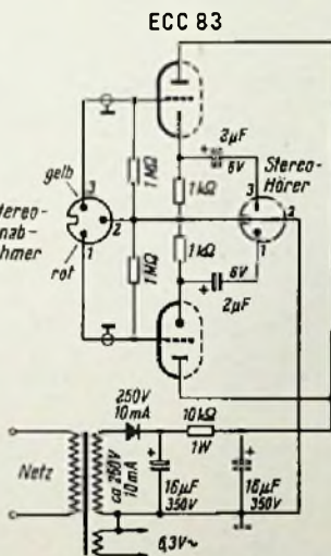
Bild 1. Schaltungen eines Stereo- und eines Normal-Kopfhörers
