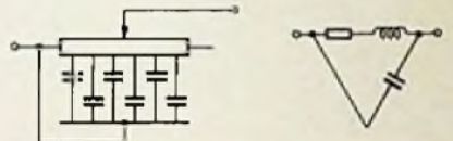
Bild 2. Abschirmung mit Anfang der Widerstandsbahn verbunden
