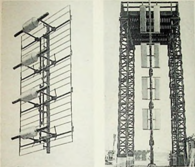
Bild 1. Bratband-Dipolfeld für Band III. Vier solche Felder bilden die Nord- und eines bildet die Südantenne des Fernsehenders auf dem Säntis
