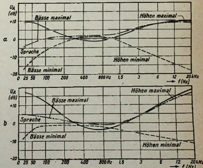
Bild 4. Wirkung der Höhen- und Tiefenregelung bzw. des Sprachschalters auf die Frequenzcharakteristik des Verstärkers a) Lautstärkenregler L auf „voll“ = 0 dB b) Lautstärkenregler L auf -40 dB
