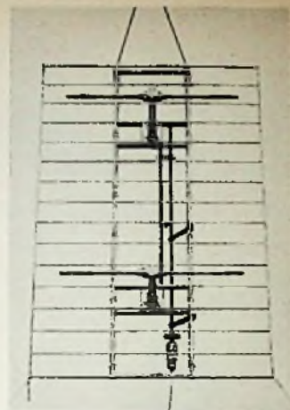
Bild 5. Breitband-Dipolfeld für UKW-Rundfunk in Band II mit Reflektorgitter
