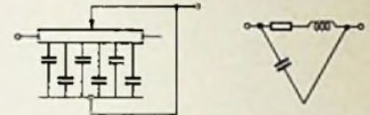
Bild 1. Abgriff des Potentiometers mit Abschirmung verbunden. Die Kondensatoren stellen die Streukapazitäten zwischen Potentiometerwicklung und Gehäuse dar
