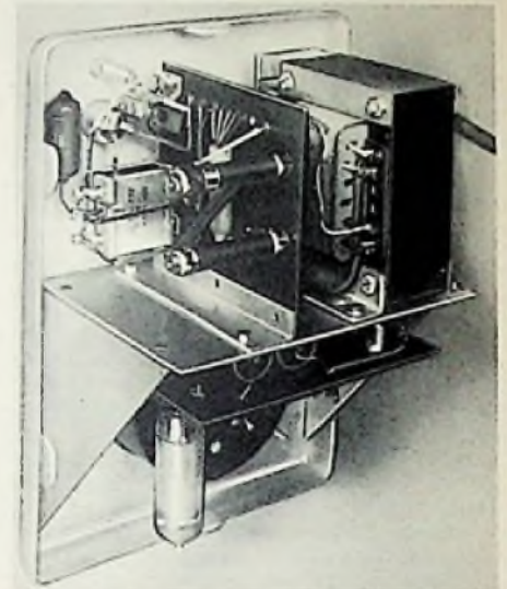
Bild 4. Unterseite des Chassis
