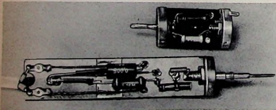
Bild 5. Innen-Anordnung des Tastkopfes und des Aufsteck-Spannungsteilers. Die Verbindungen werden durch eingelenkete Messing-Hohlknoten gehalten
