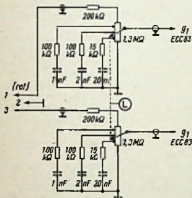
Bild 7. Die Schaltung eines gehörrichtigen Stereo-Lautstärkereglers
