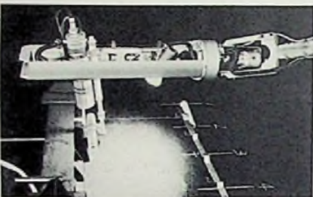
Ferngesteuerte „Hand“ mit Vidicon-Fernsehkamera für Arbeiten im Atomreaktor Windscale
