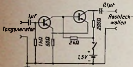
Schaltung eines Schmitt-Triggers, der vom Tongenerator gesteuert wird
