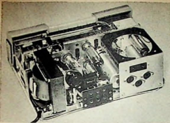
Bild 5. Blick in den Verstärker NG 5601; rechts drei Anschlüsse für Tonbandgerät, Rundfunkempfänger und Tonabnehmer, in der Mitte vorn Buchsen für die Lautsprecher
