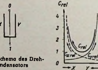
Rechts: Bild 2. Abhängigkeit der Kapazität von den Plattenabständen bzw. der Lage des Rotors
