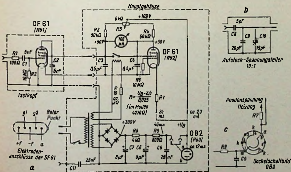
Bild 2. Gesamtschaltung; a = Anzeigeteil und Stromversorgung, b = Aufsteck-Spannungsteiler, c = Schutzschaltung zum Unterbrechen des Heiz- und Anodenkreises beim Herausziehen des Stabilisators
