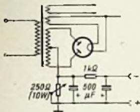
Schaltung der Ergänzung des Netzteils zur Versorgung von Transistoren
