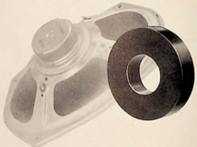
VALVO-Lautsprecher WE 73564 mit Ferroxdure-Magnet
