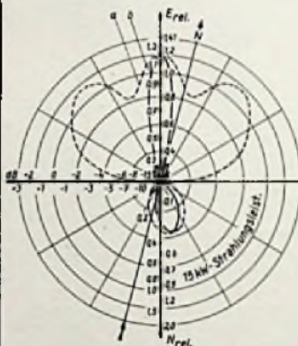
Bild 6. Strahlungsdiagramm der Fernsehantenne in Band III; a) horizontal, b) vertikal
