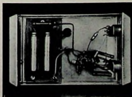
Bild 3. Unteransicht des Impedanzwandlers
