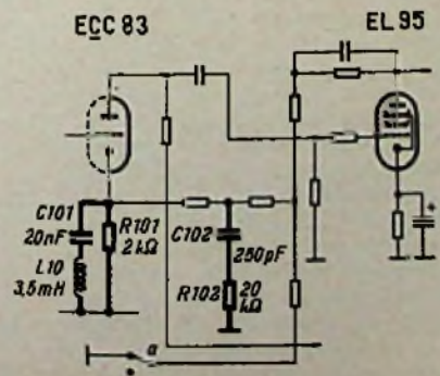
Bild 1. Die erforderlichen Änderungen der Originalschaltung sind stark eingezzeichnet
