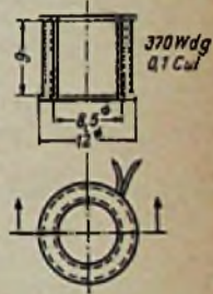
Bild 2. Bau- und Wickelskizze der Entzerrer-Drossel
