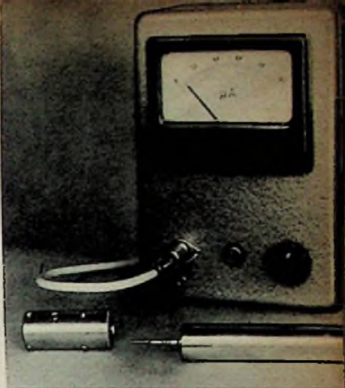
Bild 1. Ansicht des Audion-Röhrenvoltmeters
