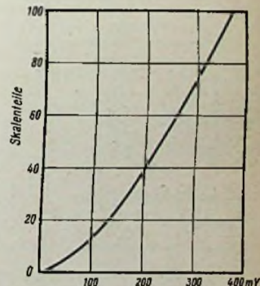
Bild 8. Eichkurve des Röhrevoltmeters. Vereinfachte Darstellung; für den praktischen Gebrauch wurde die Eichkurve auf Millimeterpapier gezeichnet
