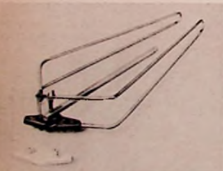
Bild 5. Neue Dachrinnen- und Fensterantenne mit V-Dipol Modell Lyra von Hirschmann zum Selbstmontieren
