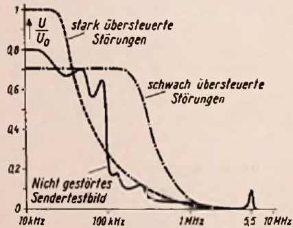
Bild 31. Schematisiertes Störpektrum, gemessen an der Video-Endstufe
