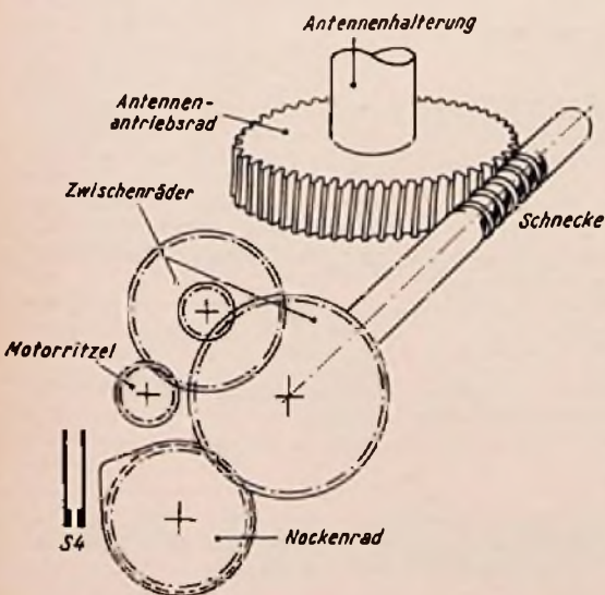
Bild 2. Schematische Darstellung des Antriebs im Antennenrotor mit dem Impulsschalter S4
