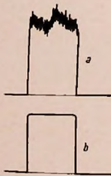
Bild 30. a = Störimpuls mit höherfrequenten Störspitzen, b = höherfrequente Störspitzen im Zf-Verstärker begrenzt
