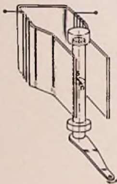
Bild 5. Bei dem neuen magneto-dynamischen System von Philips induziert ein quer-magnetisierter Fer-roxdure-Stab die Tonspannungen in den Spulen auf einem Weicheisen-kern
