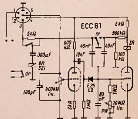
Bild 9. Schaltung des Acustomat D für automatische Dia-Projektion
