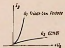
Bild 37. Überlegenheit der Gitterstromkennlinie am Gitter 3 der ECH 81 gegenüber der Gitterstromkennlinie einer Triode oder Pentode für die Abtrennung
