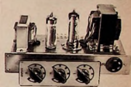
Bild 2. Phono-Bar-Verstärker in Chassis-Ausführung (Klein & Hummel)
