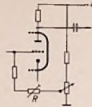
Ein Wackelkontakt an R läßt die Zeilenfrequenz springen
