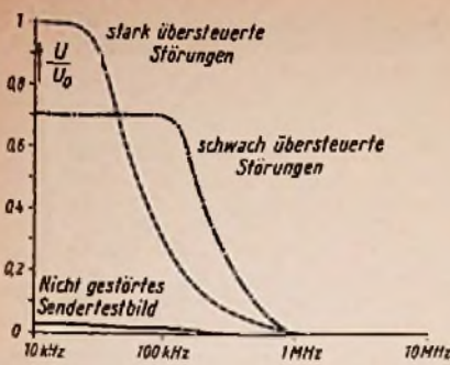
Bild 32. Schematisiertes Störpektrum an der Anode des Störinverters
