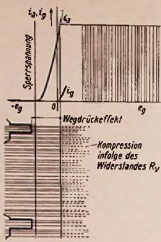
Bild 28. Häufige Störungen drücken das Synchronsignal aus dem Abtrennbereich der Abtrennstufe
