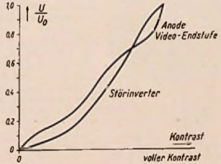
Bild 35. Ausgangsspannung der Videostufe und des Störinverters in Abhängigkeit vom Kontrast bei einem bestimmten künstlichen Störorgang gemessen
