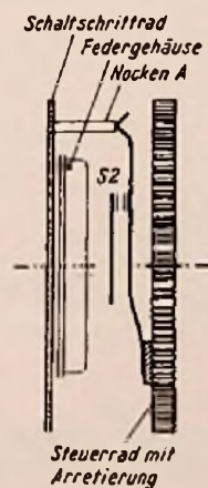
Bild 4. Zusammennocken von Steuerrad und Schaltschrittrad im Kommandogerät
