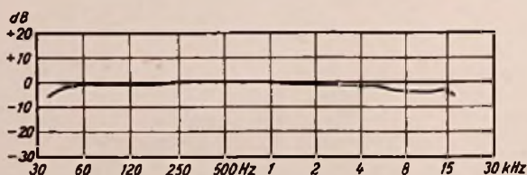
Bild 7. Frequenzgang des keramischen Tonabnehmersystems 3 TS (Telefunken). Die Kapsel wurde an einen Entzerrier-uerstärker mit einem Eingangswiderstand von 840 kΩ über ein Meßkabel von 360 pF Kapazität angeschlossen
