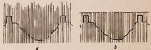
Bild 26. Zündstörungen auf dem Videosignal, a = unbegrenzt, b = begrenzt und abgeschnitten
