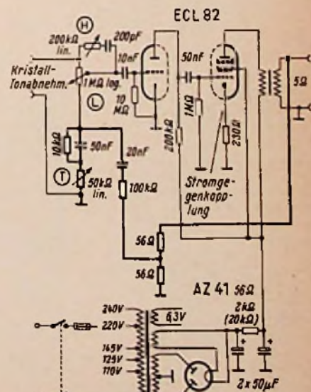
Bild 3. Schaltung eines Phono-Bar-Verstärkers
