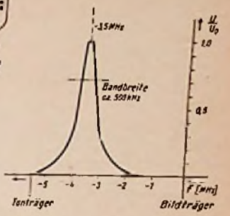
Bild 34. Frequenzgang des Stör-Inverters
