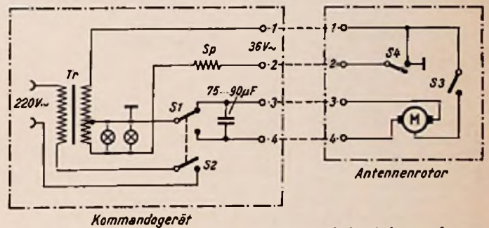
Oben: Bild 3. Schaltung von Kommandogerät und Antennenrotor
