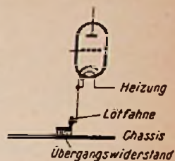
Der Heizstrom ergab an dem Übergangswiderstand der Lötöse gegen das Chassis einen Wechselspannungsabfall, der in den Katodenkreis eingekoppelt wurde
