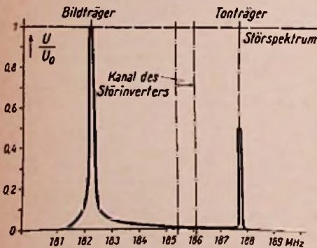
Bild 29. Schematisiertes hochfrequentes Spektrum des Sendertestbildes und einer Funkstörung
