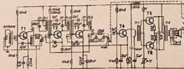
Bild 2. Schaltung des Taschensupers Sony
