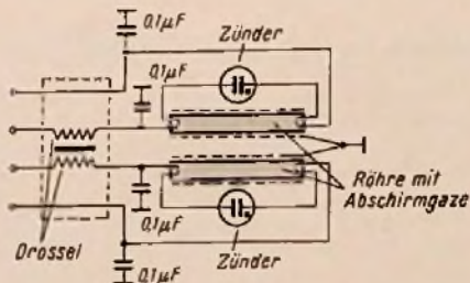
Prinzipschaltung einer Leuchtstoffröhre mit abgeschlossener Abschirmung
