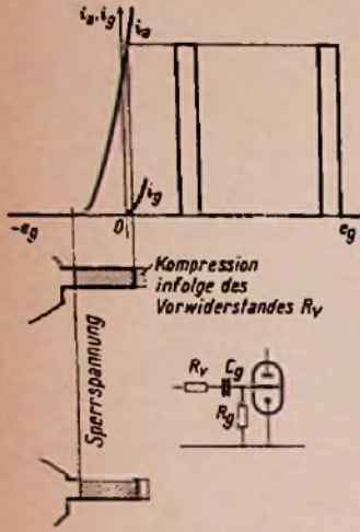
Bild 27. Arbeitsweise der Impuls-Abtrennstufe
