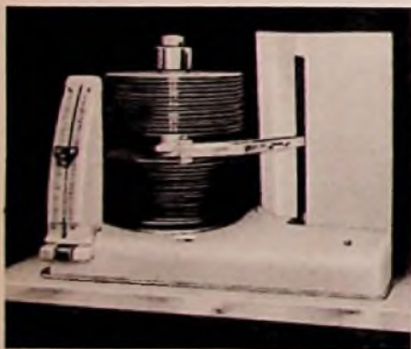
Bild 6. Ein Tonarm mit zwei Abtastsystemen kann in diesem Wechsler je nach Programmeinstellung Ober- oder Unterseite jeder beliebigen Platte aus einem Stapel von 30 Stück abtasten (Wiegandt)
