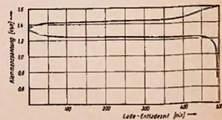
Rechts: Bild 2. Spannungsverlauf bei Ladung und Entladung eines Nickel-Cadmium - Sammlers vom Typ FSG 8
