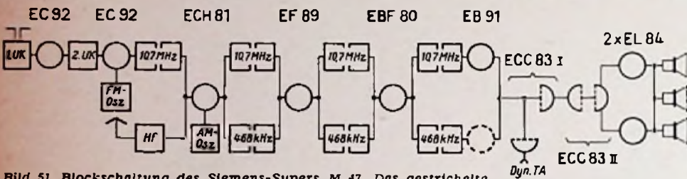
Bild 51. Blockschaltung des Siemens-Supers M 47. Das gestrichelte Röhrensystem hinter dem letzten AM-Zf-Filter gehört zur Röhre EBF 80 (Diode)
