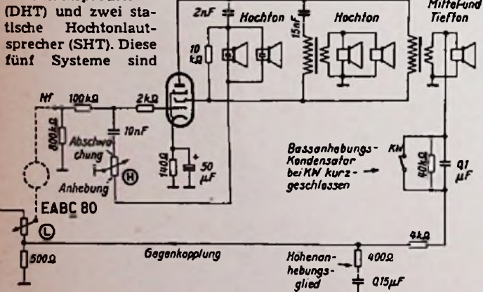
Bild 59. Ankopplung der Lautsprecher beim Concertino TS
