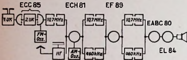
Bild 57. Blockschaltung Jubilato 55
