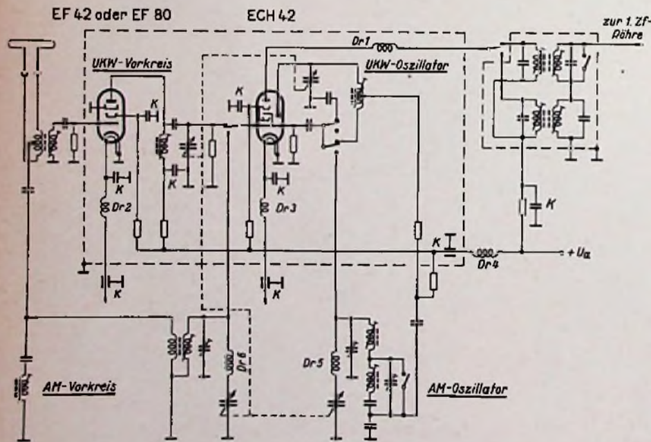
Bild 1. Schaltbeispiel eines entstörten UKW-Aufbauteiles. Die mit K bezeichneten Kondensatoren sind unbedingt in Keramik-Ausführung zu wählen. Die Spulen Dr 1 bis Dr 4 bestehen aus 20 Wdg. 0,5 mm CuL, 5 mm \varnothing . Die Spulen Dr 5 und Dr 6 bestehen aus 6...10 Wdg. 0,5 mm Schaltdraht, 5 mm \varnothing . Man erkennt, über welche Leitungen die Störstrahlung verschleppt werden könnte, was aber durch die sorgfältige Verblockung und Verdrosselung verhindert wird. Unter Umständen ist es zweckmäßig, den Parallel-Kondensator des ersten 10,7-MHz-Bandfilterkreises unmittelbar hinter der Drossel Dr 1 an Masse anzuschließen
