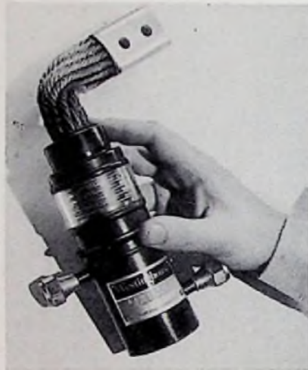
Wassergekühlte Hochleistungs-Gleichrichterdiode mit Germanium, hergestellt von der Westinghouse Electric Corporation
