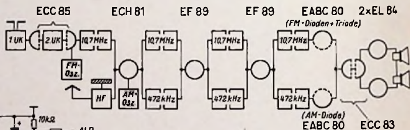
Bild 52. Blockschaltung Tekade W 488
