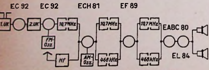
Bild 49. Blockschaltung des Siemens-Supers C 40
