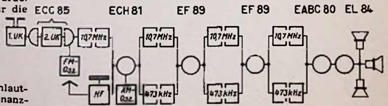
Bild 60. Blockschaltung des Wega-Prominent
