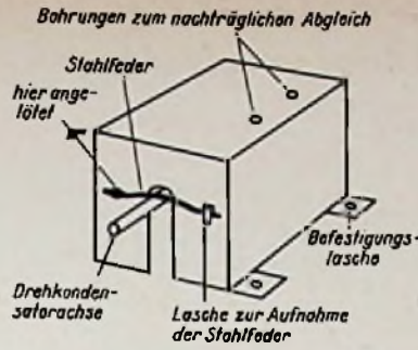
Bild 3. Abschirmkästchen. Innerhalb des Kästchens befindet sich der UKW-Teil mit dem kombinierten Drehkondensator. Um Röhrenwechsel zu ermöglichen, wird der Abschirmkasten mit Befestigungslaschen mit dem Gerätechassis verschraubt.
