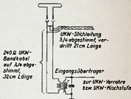
Bild 2. UKW-Eingang mit Stichleitung. Die Stichleitung wird auf einen Dorn von ca. 10 mm \varnothing aufgewickelt, dadurch wird sie breitbandiger und unterdrückt die Störstrahlung über den Bereich hinweg gleichmäßiger
