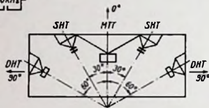
Bild 58. Lautsprecheranordnung beim Concertino TS
