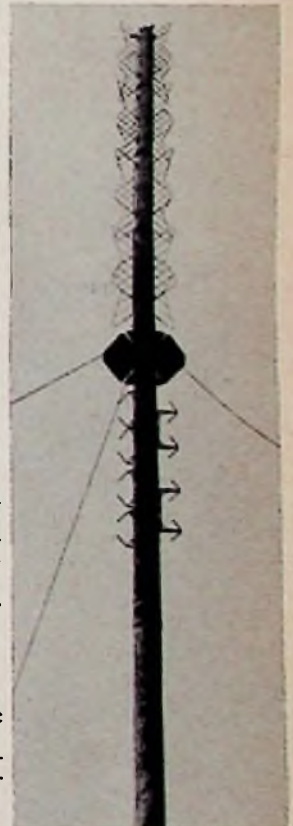
Bild 1. Vierfach-Schmetterlingsantenne mit Antennengewinn 4 für Rundstrahlung (oben); unter dem Eisabwischer die UKW-Antenne des UKW-Rundfunksenders, bestehend aus drei Zweierfeldern mit geknickten Dipolen
