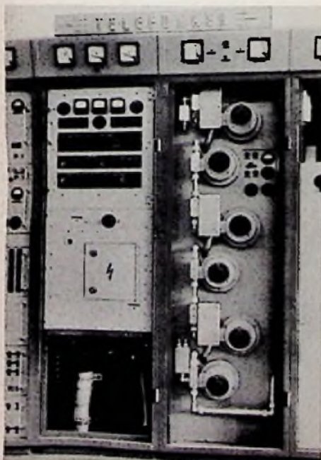
Links: Bild 2. Schalttableau (links) und Restseitenbandfilter
