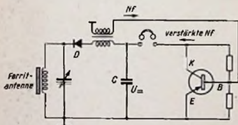
Mit „freier Energie“ gespeiseter Transistorempfänger
