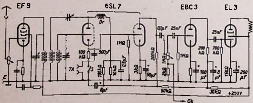
Auch von einem Katodendetektor läßt sich auf den Gitterkreis rückkoppeln
