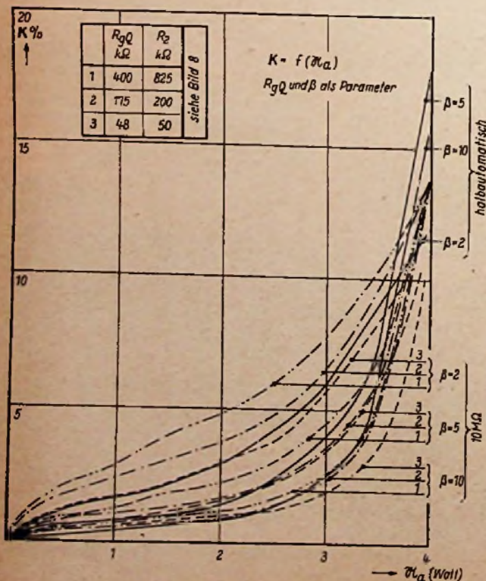
Bild 9. Klirrfaktorcurven der Telefunken-Röhren EABC 80 und EL 41
