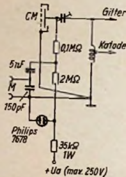
Bild 2. Abgeänderte Eingangsschaltung für äußere Tonnspannungsquellen
