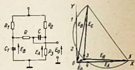
Bild 4. Erweiterte RC-Schaltung nach Sulzer
