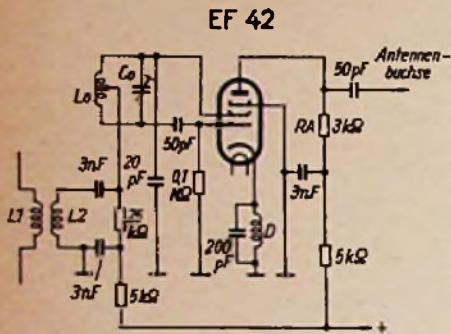
Schaltung des UKW-Super-Vorsatzgerätes
