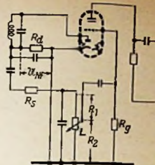
Bild 8. Prinzip-Schaltung zur Berechnung des Widerstandes R_g .
