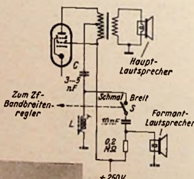
Bild 2. Ansteuerung des Formant-Lautsprechers an die Spule L der 9-kHz-Sperre
