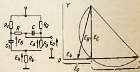
Bild 5. Wirkung des Fußpunktwiderstandes für eine Schaltung nach Bild 4
