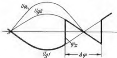
Bild 11. Gitterspannungsverlauf (dick ausgedr.) bei einer Sprungsteuerung unter Verwendung einer Drossel mit geknickter Magnetisierungskennlinie nach Bild 10
