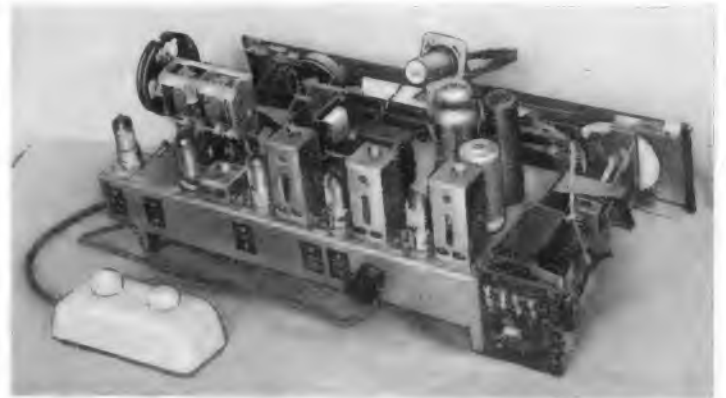
Chassis des Loewe-Opta-Atlas mit FernbedienungskdStchen
