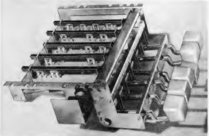
Ansicht eines sechsstelligen Drucktasten-Aggregates
