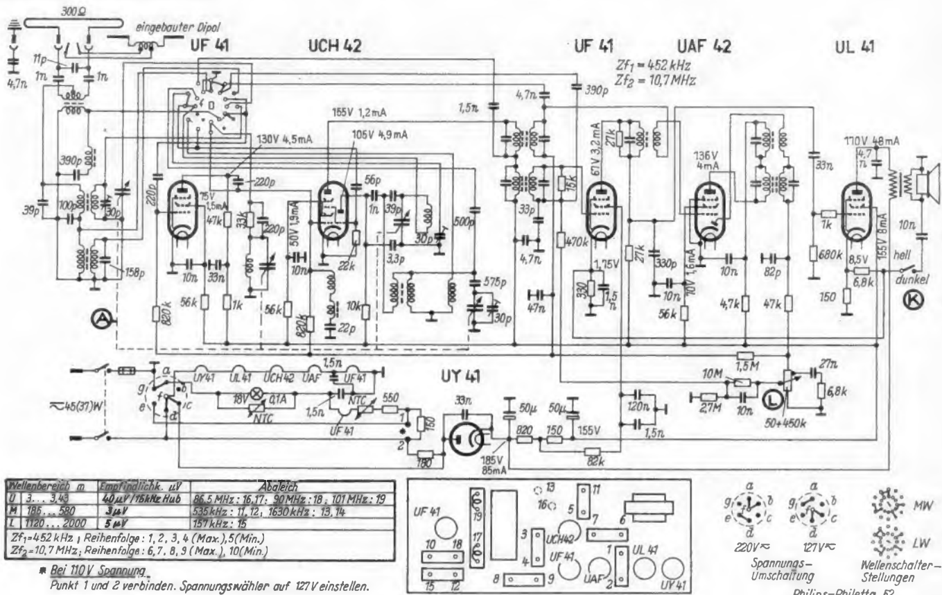
Schaltung der Philetta 52
