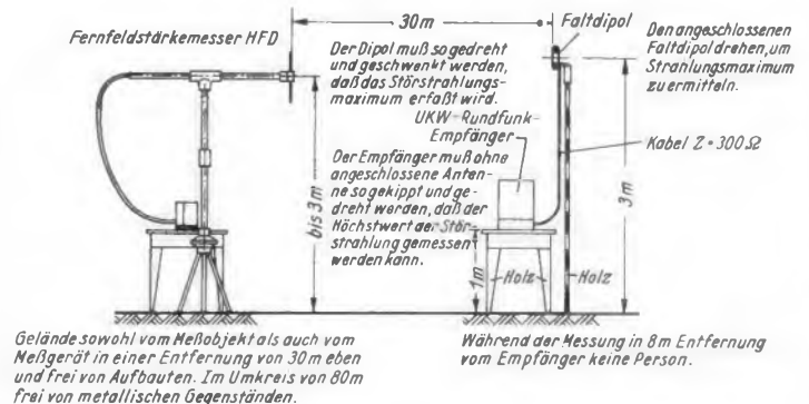
Bild 2. Störfeldstärke-Meßanordnung für UKW-Rundfunkempfänger
