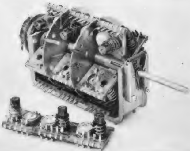
Görler-Spulenrevolver
