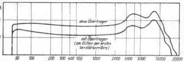
Unten: Frequenzgang des Ronette-Zellenmikrofons Typ R 572 L ohne und mit Übertrager
