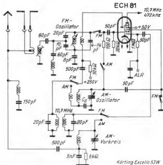
Triodensystem einer ECH 81 als UKW-Mischröhre mit dem Heptodensystem als 1. Zf-Verstärkerstufe für FM
