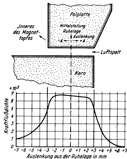
Bild 2. Verlauf der Kraftflußdichte im Luftspalt und in der Umgebung des Luftspaltes bei den darüber angedeuteten Abmessungen von Polplatte und Kern
