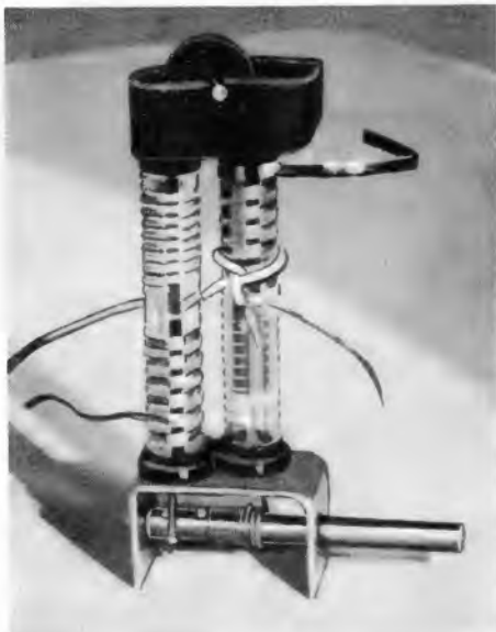
Bild 1. Ansicht des UKW-Doppelvariometers mit Folienwicklung
