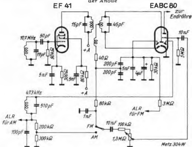
Verbundröhre EABC 80 in FM- und AM-Demodulatorschaltung und als 1.1-Verstärkerstufe
