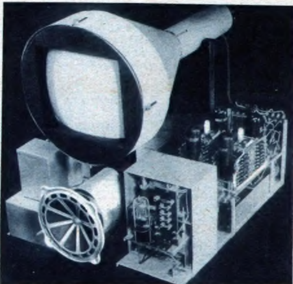
Hier einmal wieder das Innere eines modernen Fernsehers mit seinen vielen komplizierten Einheiten. (Werkphoto DS. Loewe)
