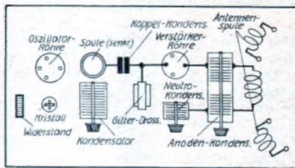
Aufbauplan eines selbstregerten Senders (Colpitts) und eines zweistufigen fremdgeführten Senders (Kristall-Oszillator mit neutralisierter Eingitter-Röhre).
