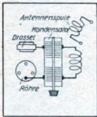
Aufbauplan eines selbstregerten Senders (Colpitts) und eines zweistufigen fremdgeführten Senders (Kristall-Oszillator mit neutralisierter Eingitter-Röhre).
