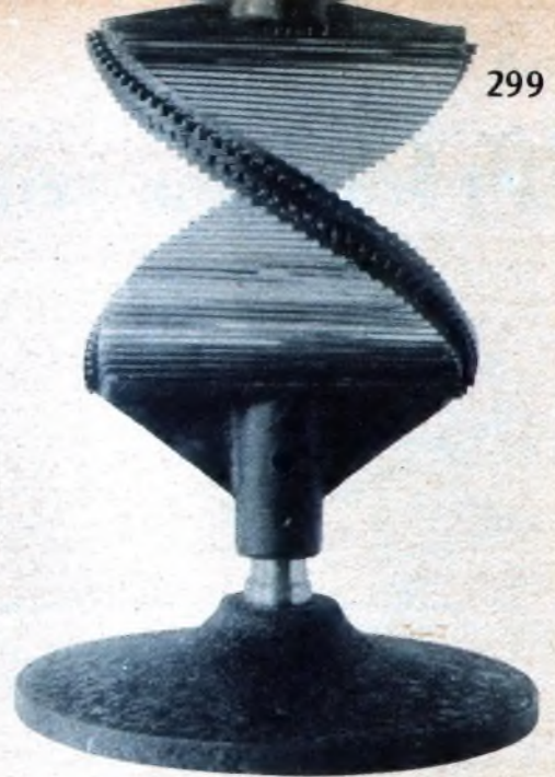
Die Fa. Tekade zeigte wieder ihren Spiegelrad-Empfänger, den einzigen noch vorhandenen mechanischen Empfänger. Seine Aussichten scheinen uns noch nicht erloschen. Die Qualität der Bilder ist ausnehmend gut. (Werkphoto)
