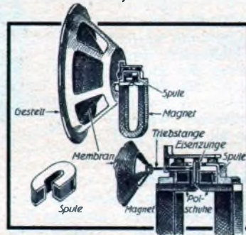
Ein magnetischer Lautsprecher. Links oben das Gestell mit vollkommener Ausrüstung. Links unten die im angeschnittenen Zustand dargestellte Spule. Sie ist fest angeordnet und steht demgemäß nicht mit der Membran in Verbindung. Rechts unten die beiden Pole des Dauermagneten mit den Polschuhen. Auf ihnen die Spule. — Die Eisenzunge ist an ihrem oberen Ende ganz dünn, so daß sie schwingen kann. An ihr ist die Triebstange befestigt, die die Verbindung mit der Membran des Lautsprechers herstellt. Um sie sicher zu führen, ist sie durch einen dünnen Blechstreifen, die „Geradführung“, gehalten.
