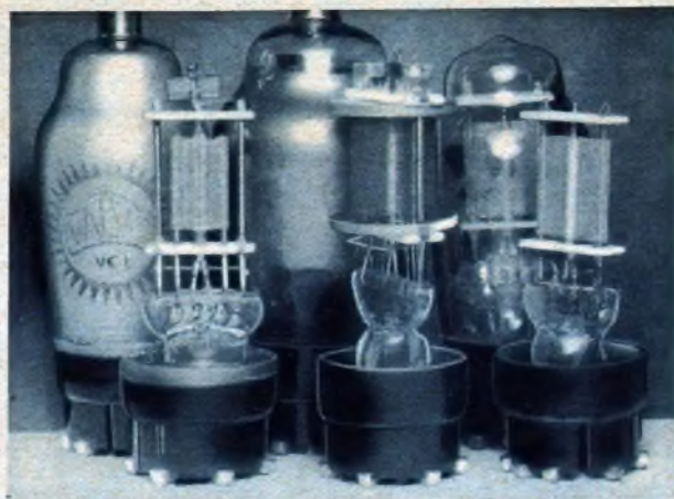
Eigentlich schade, daß das Wunderwerk der Röhre unsichtbar im Innern des Glaskolbens verdrillt liegt. (Volksempfänger-Röhren für 55-Volt-Heizung). Werkfoto Valvo.
