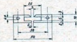
Abb. 2. Die beiden Polschuhe und ihre Abmessungen.
