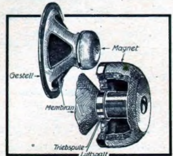
Der dynamische Lautsprecher hier mit permanent-dynamischem System; das Magnetfeld wird also durch einen Dauermagneten erzeugt. Dieser sitzt hinten auf dem Gestell. Zwischen Mittelbolzen und vorne befindlichem Deckel ein Luftspalt, in den die Triebstange hineintaucht. Die Spule sitzt auf einem Ansatz der Membran und ist daher in der Lage, die Membran direkt anzutreiben. Damit sie im Luftspalt nicht streift, befindet sich am vorderen Ende des Bolzens eine „Zentrierung“.
