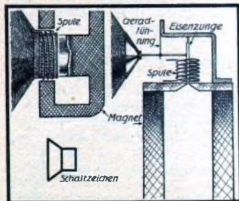
Die wesentlichen Teile des magnetischen und dynamischen Lautsprechers einander gegenübergestellt. Wir erkennen in beiden Bildern die Spule und den Magneten. Beim dynamischen Lautsprecher sitzt die Spule fest auf dem Membranfortsatz. Beim magnetischen Lautsprecher ist die Spule an dem Magneten befestigt, während die Eisenzunge beweglich ist, deren Bewegungen durch eine Triebstange auf die Membran übertragen werden.
