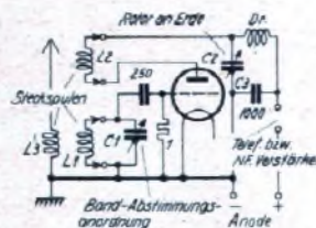
Abb. 1. Die einfachste Kurzwellenschaltung: Das Audion mit kapazitiver Rückkopplung.
