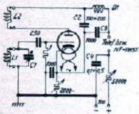
Abb. 2. Die günstigste Anordnung mit einer Dreipolröhre. Die Regelung der Rückkopplung erfolgt durch einen veränderlichen Anodenwiderstand.
