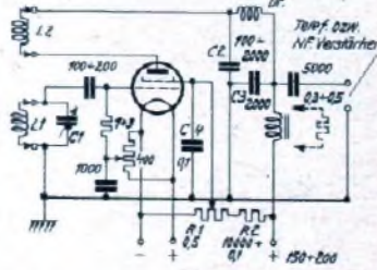
Abb. 3. Wohl die empfindlichste Schaltung: Das Vierpolröhren-Audion mit Drosselkopplung. Die Rückkopplung wird durch die Schirmgitterspannung eingestellt.
