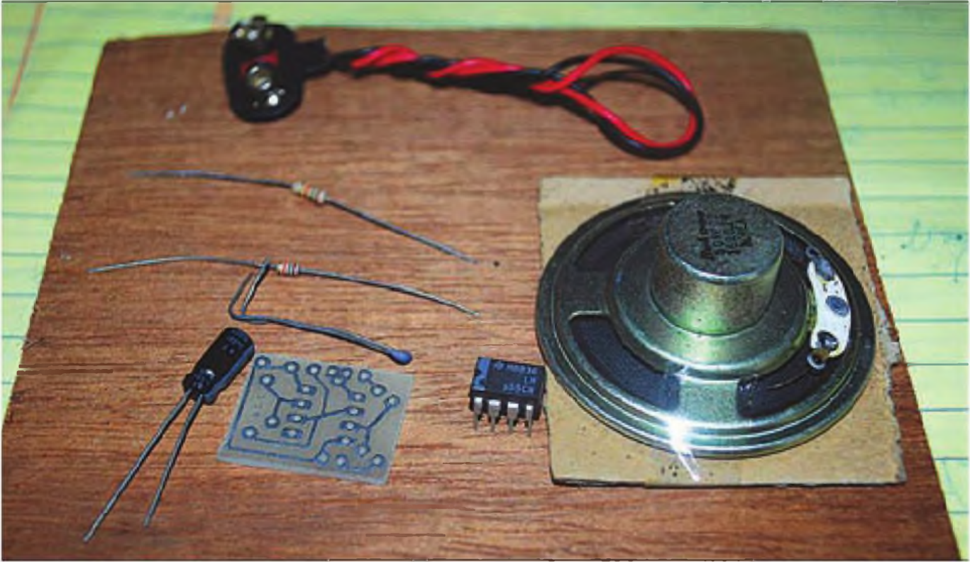
Foto B: Los componentes del kit OSC-2.
