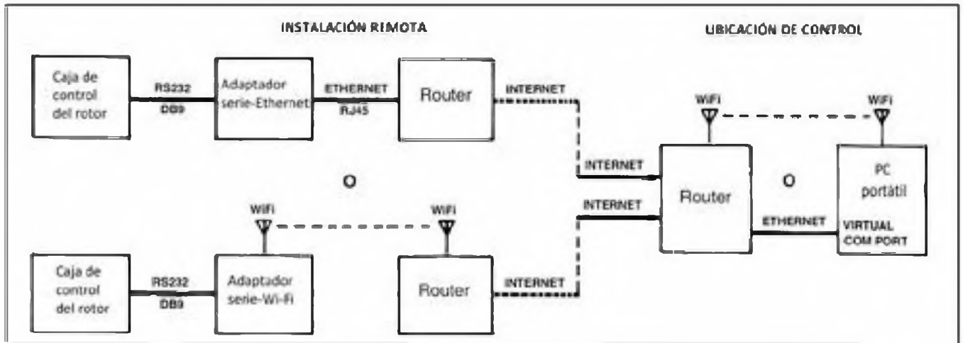
Figura 1: Dos soluciones para controlar remotamente los rotors.
