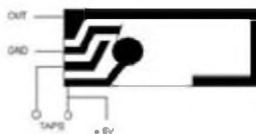
Figura 4. La conexión OUT del pulsador de contacto se conecta a la entrada del PIC.
