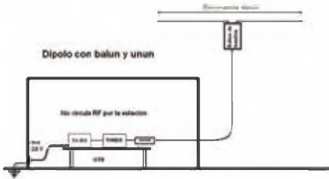
Figura 8: Dipolo con balun y con unun en la estación
