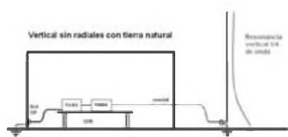
Figura 11: Vertical con tierra natural
