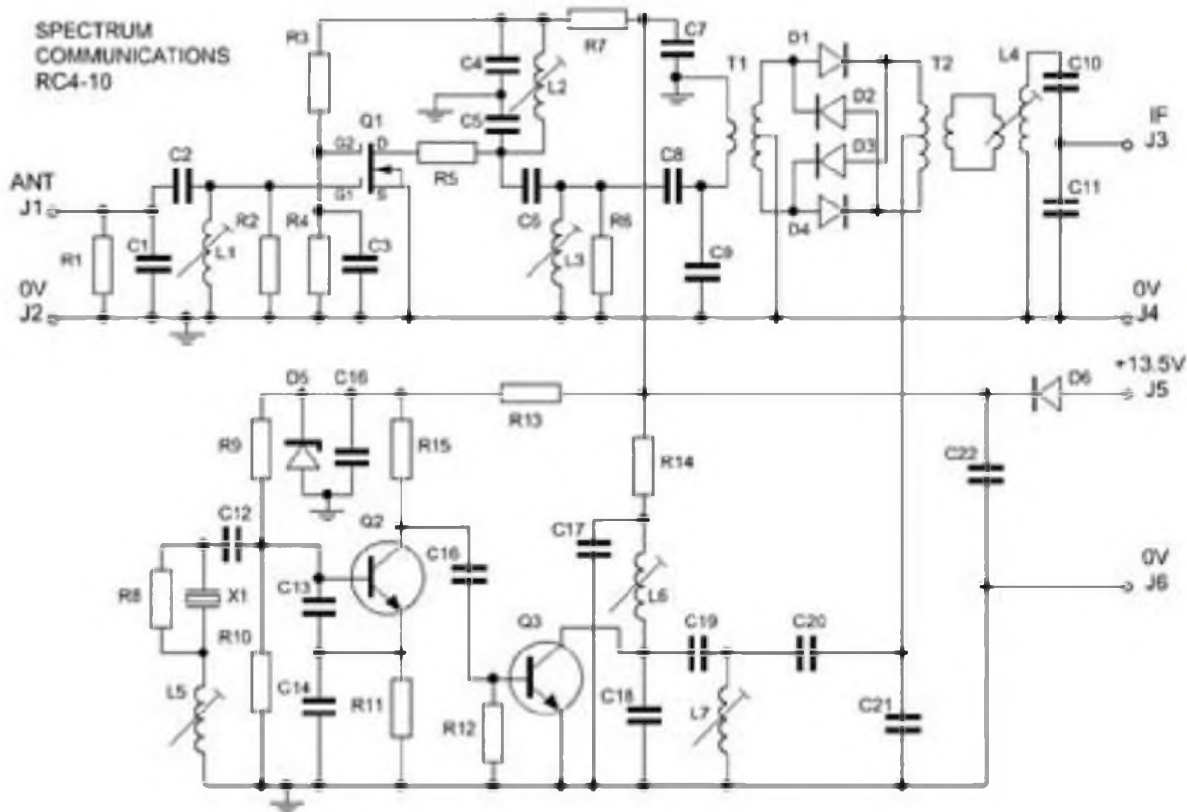
Esquema del conversor RC4-10
