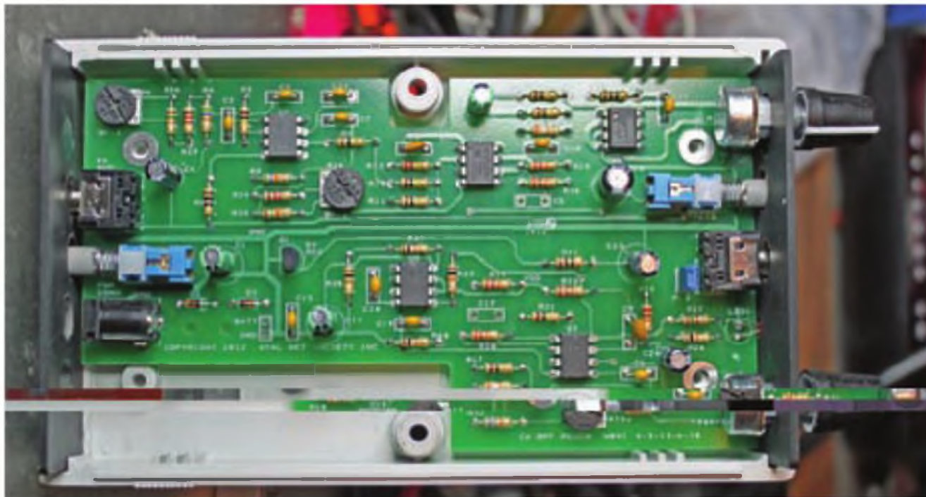
Foto A. El CW Scrubber en su caja. Sus mandos van soldados directamente a la placa del circuito.
