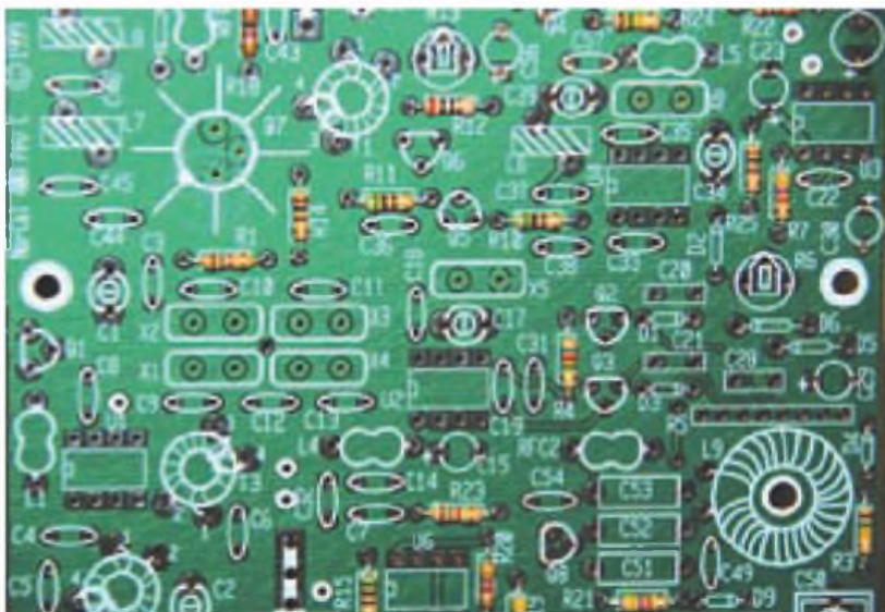
Foto B. Una vista parcial ampliada de la placa de de circuito impreso. Si consigues llenarla de componentes, el transceptor funcionará a la primera: lo prometo.
