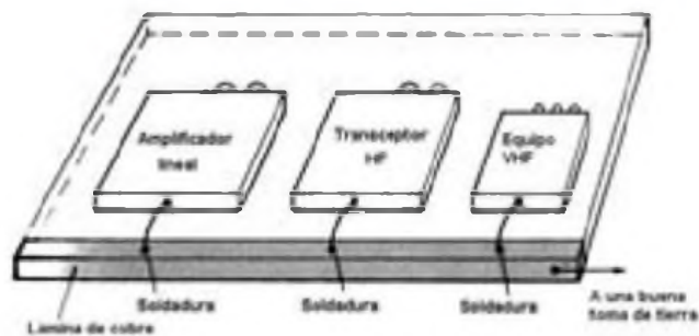
Figura 4: Puesta a tierra común de los equipos
