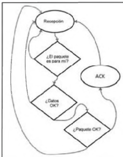
Figura 1: Un diagrama de flujo simplificado que muestra el proceso ARQ (Automatic Repeat Request = Petición automática de repetición) de un enlace de radiopaquete AX.25 desde el punto de vista del receptor. A menos que el paquete sea totalmente correcto para la estación receptora, es decir sin errores, y sea el siguiente paquete de la secuencia, no recibirá el ACK (ACKnowledge = acuse de recibo). Cuando el transmisor no recibe un ACK en un tiempo determinado, reenvía el paquete y lo repite hasta que consiga el ACK o se supere el número máximo de repeticiones admitido.
