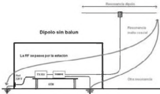
Figura 1: Dipolo sin balun y toma de tierra interior
