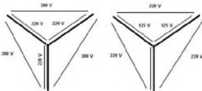
Figura 2: Redes de distribución eléctrica de baja tensión
