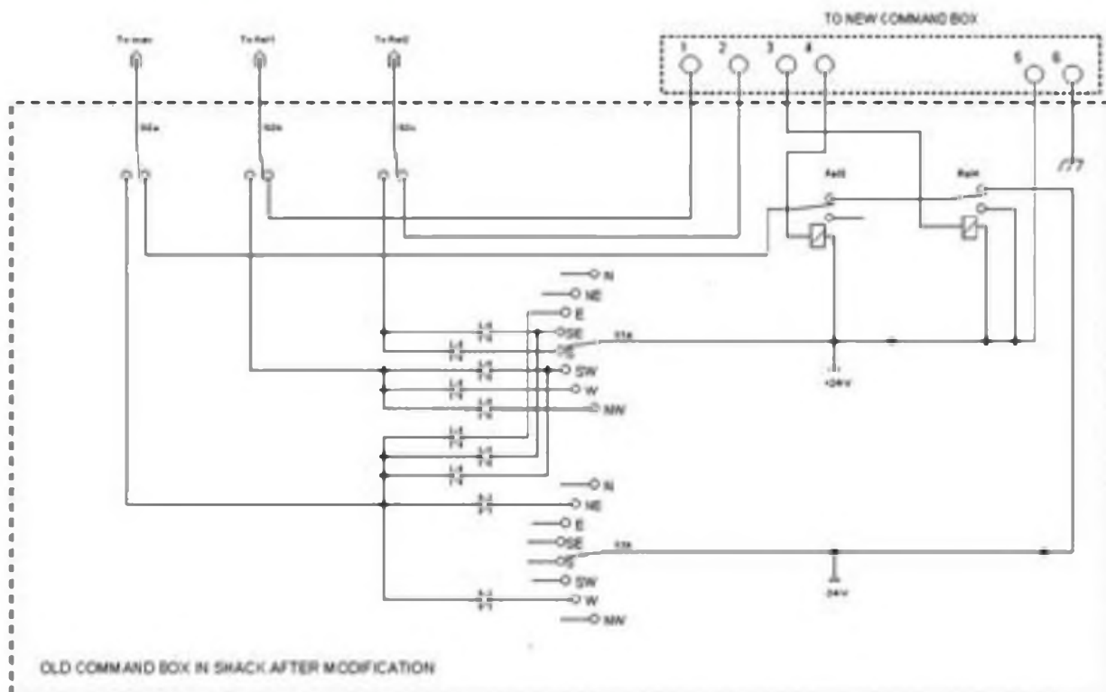
Figura 3. Esquema de la antigua caja de conmutación modificada.
