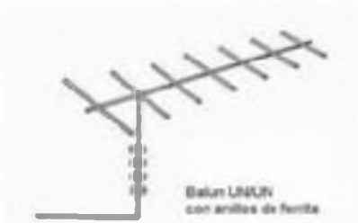
Figura 7: Unun de ferritas
