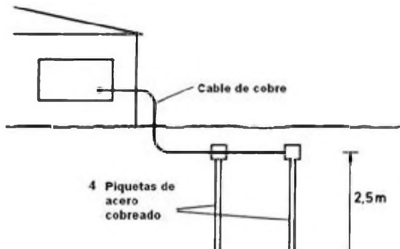
Figura 15: Toma de tierra efectiva con 4 picas
