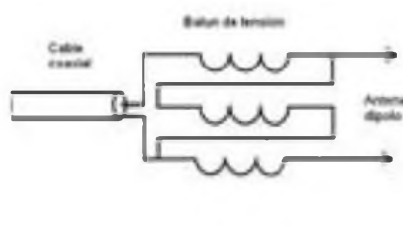
Figura 6: Balun de tensión
