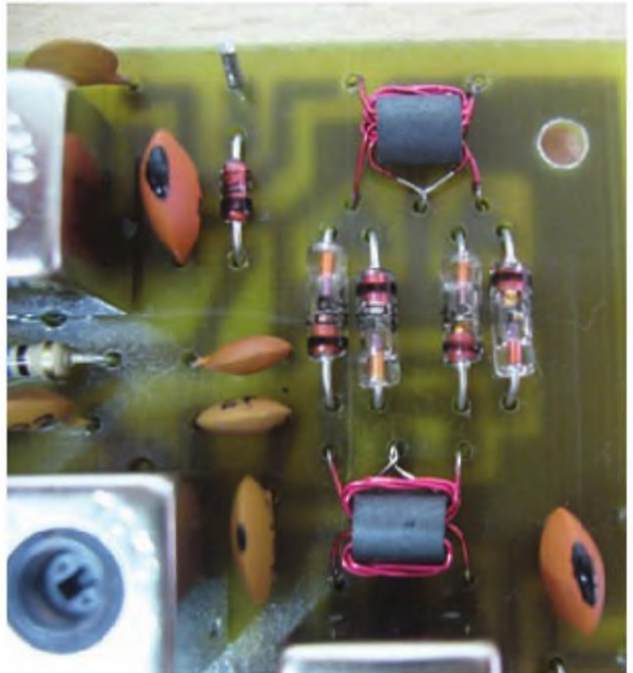
Mezclador doblemente balanceado a diodos
