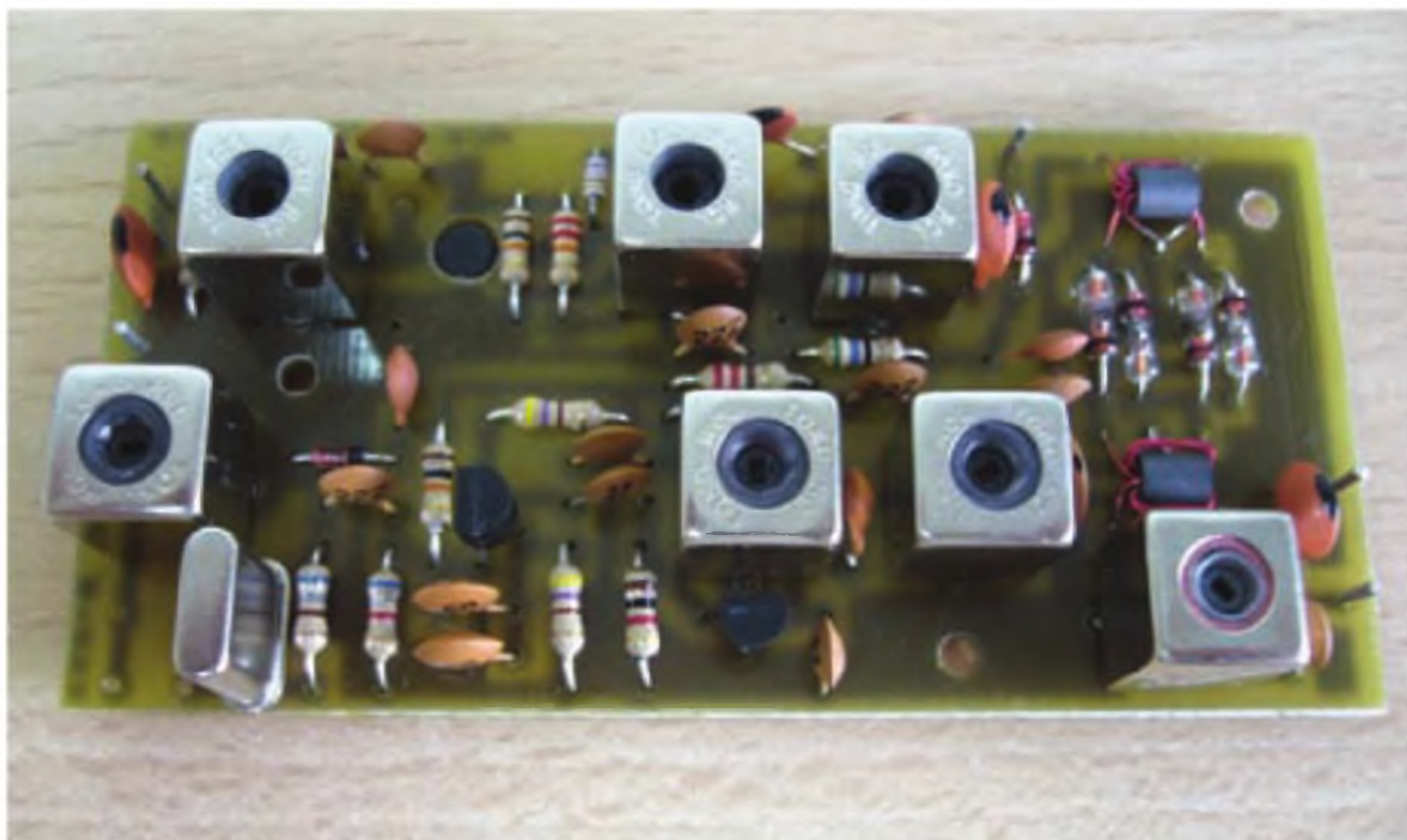
El conversor RC4-10 montado
