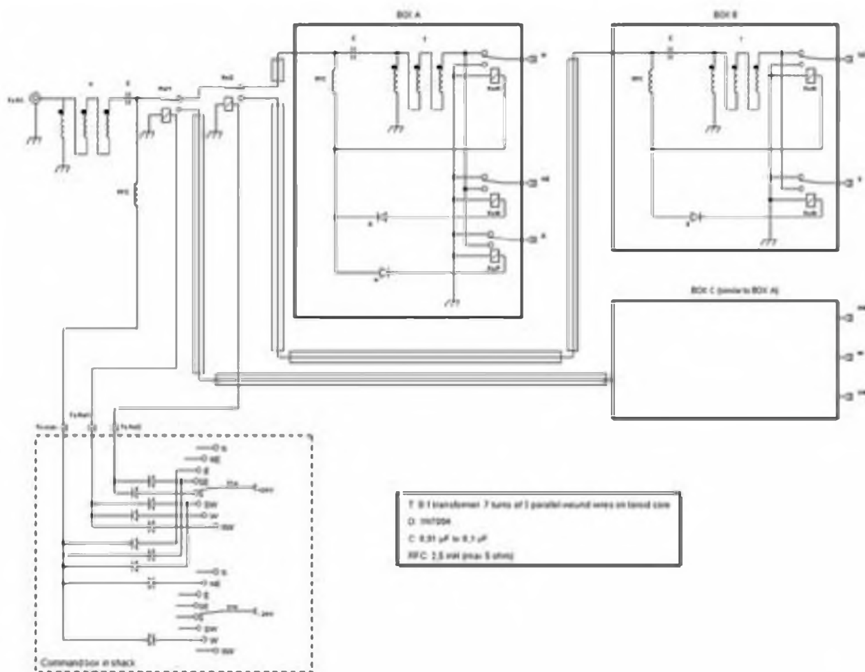
Figura 1. Mediante los relés REL1, REL2 y la tensión en el centro del cable coaxial, seleccionamos una de las ocho antenas mediante los circuitos A, B y C.
