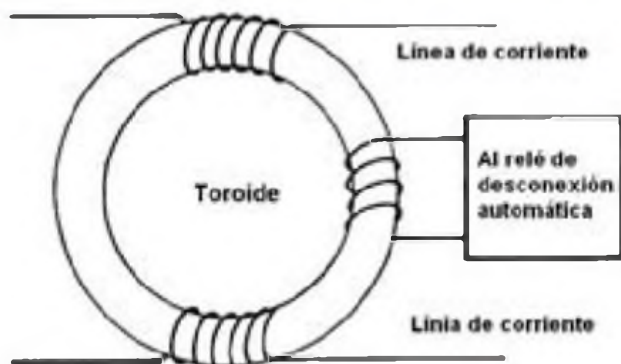
Figura 3: Esquema de un IPC o protector diferencial
