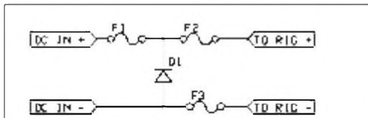
Figura 2. Otro esquema con un diodo que utiliza uno con menores especificaciones y que no ocasiona una caída de tensión a su través. Este es el circuito que prefiero.
