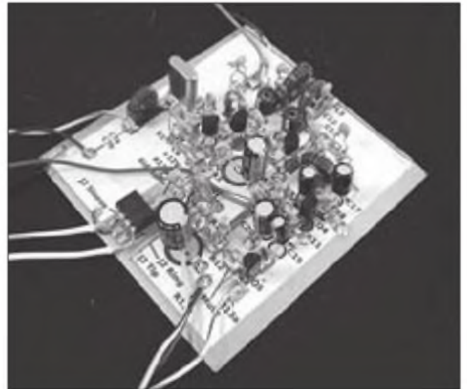
Foto A. El versátil receptor VRX-1, que puede ser montado para cualquier banda desde 160 a 10 metros, viene con un diagrama de montaje dibujado sobre la placa y es un buen kit para iniciarse en el montaje estilo Manhattan.
