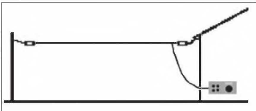
Figura 2. La clásica antena de hilo largo. Esta puede tener cualquier longitud de cable. Por supuesto que necesitarás algún tipo de acoplador entre el cable y el transmisor para adaptar la impedancia en las diferentes bandas y una toma de tierra como contraantena (falta en la ilustración).
