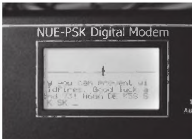
Foto E. "Sólo tú puedes evitar los fuegos", es el lema del Oso Smokey.
