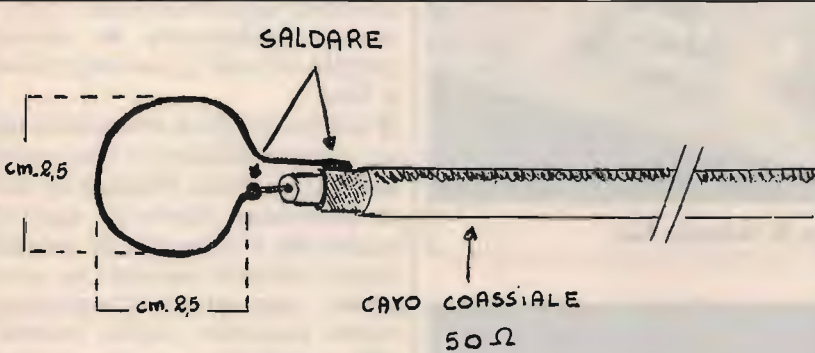
Sonda da collegare al frequenzimetro.
