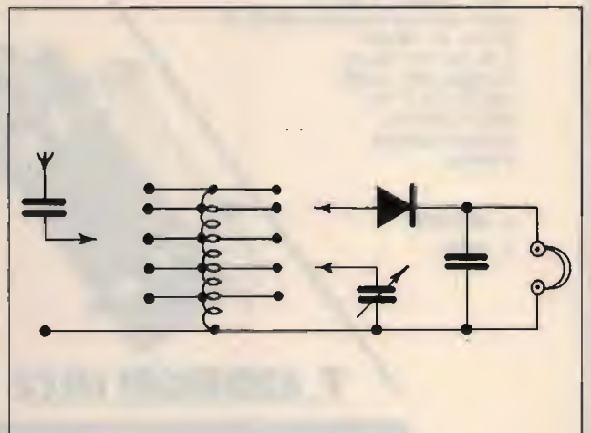
figura 2 Galena modificata per ricevere più stazioni: funzionava più che altro da adattatore di impedenze.
