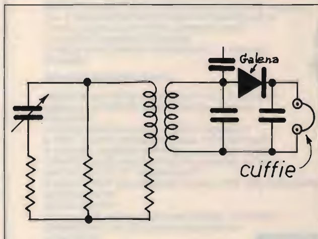
figura 1 La prima galena: malgrado il malloppo ozioso costituito dal circuito equivalente di antenna (parte a sinistra), funzionava benissimo negli anni '20. Solo col crescere delle Emittenti evidenziò i suoi difetti.
