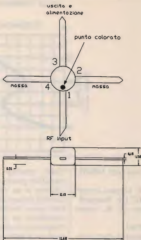
Dimensioni tipiche e piedinatura di un MMIC.
