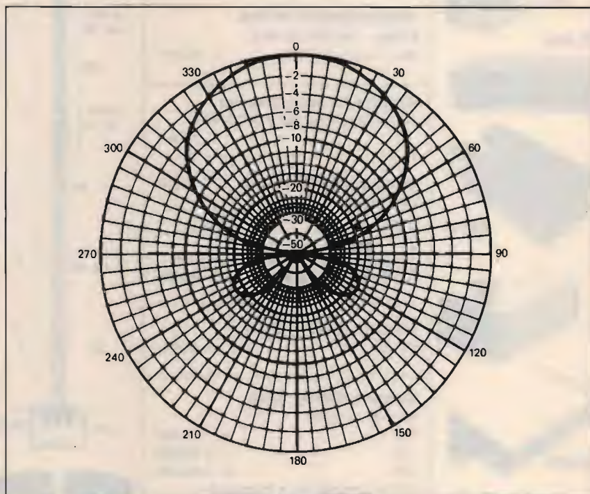
figura 1 Diagramma teorico di irradiazione di una cortina di loop.
