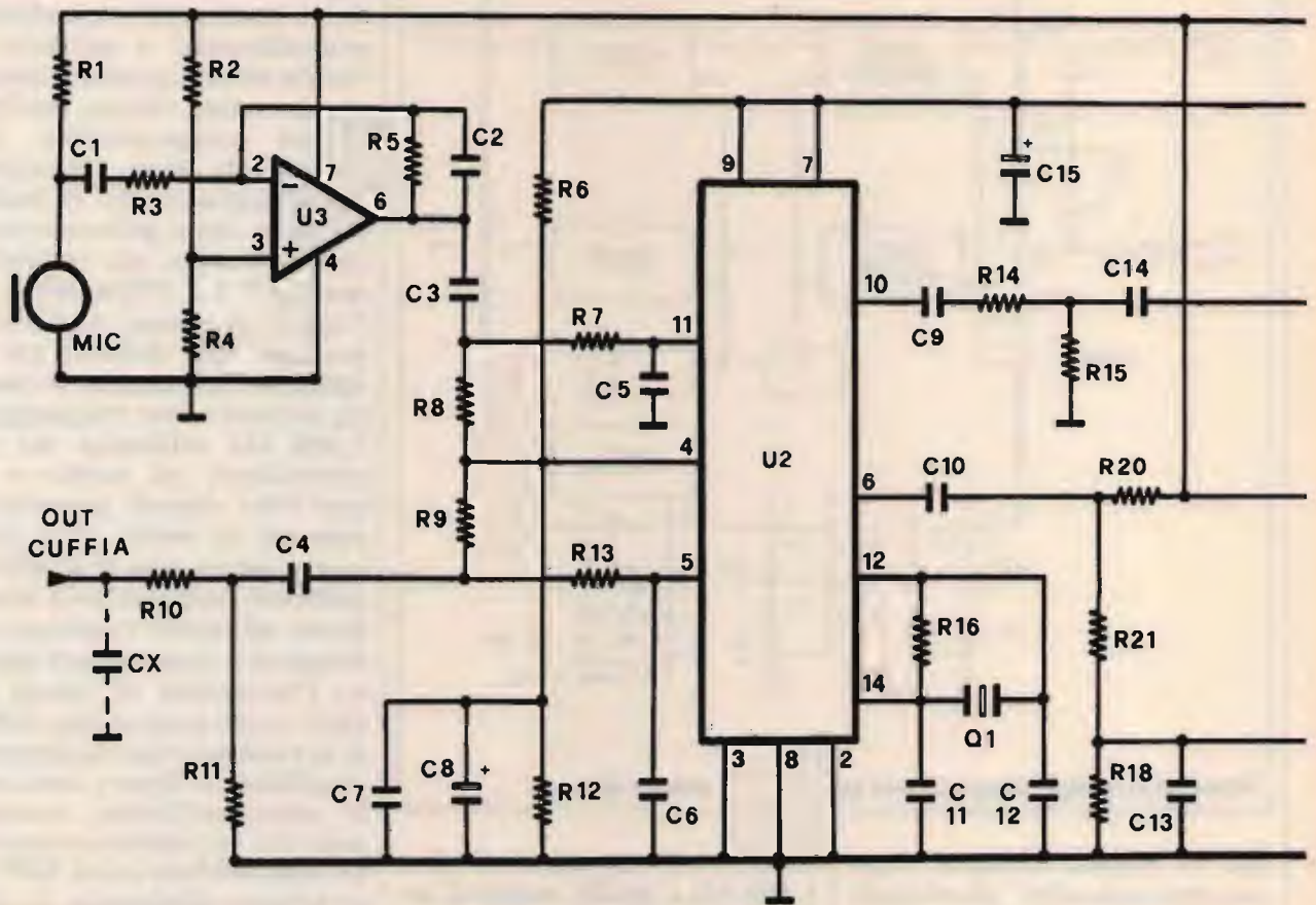
Schema elettrico.
