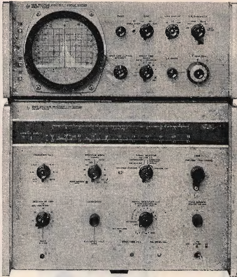
figura 5 Spectrum analyzer 8551B/851B della Hewlett-Packard. È il tipico analizzatore di spettro inteso universalmente come tale. Presenta un campo di frequenza da 10 MHz a 42 GHz. Dinamica sul tubo RC: 60 dB. Campo di frequenza massima visualizzazione sul tubo RC: 2.000 MHz.
