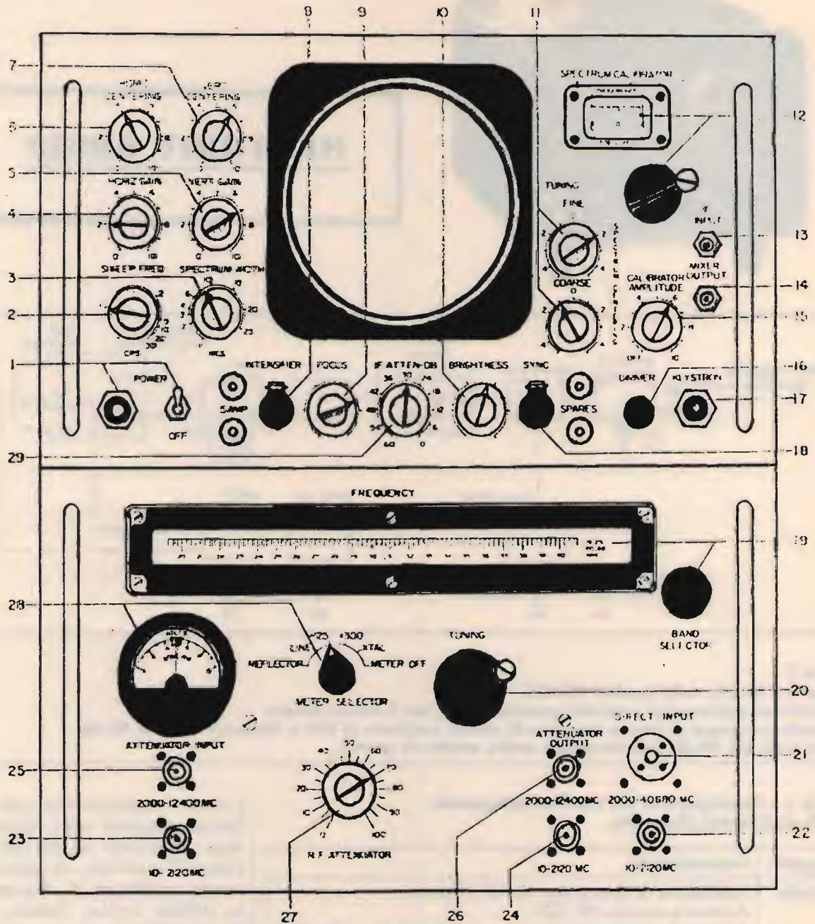
figura 3 L'analizzatore TS-1010/UPM-84.
