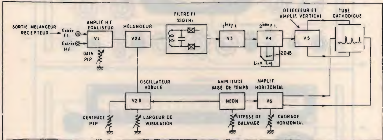
figura 2 Schema a blocchi dell'Heathkit SB-620. È questo un apparecchio costruito appositamente per il radioamatore. Presenta un campo di sweep massimo di alcune centinaia di kHz e dinamica di 20 o 40 dB. Nella scala dei 40 dB può consentire anche analisi di spettro.
