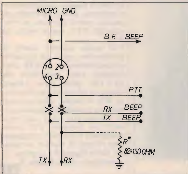
figura 4 Schema di cablaggio del Roger-beep all'Alan 48.
