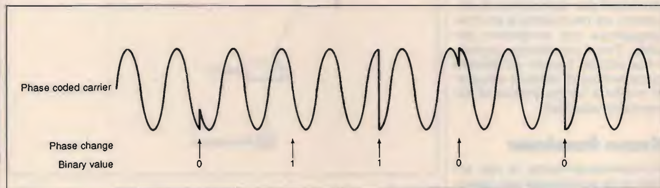
figura 2 Lo standard di gruppo 3 usa la modulazione PSK, in cui il valore 0 o 1 dei singoli bit dipende dal valore del bit precedente e dal cambiamento di fase. Dall'alto al basso: portante codificata in fase; cambiamento di fase; valore binario.
