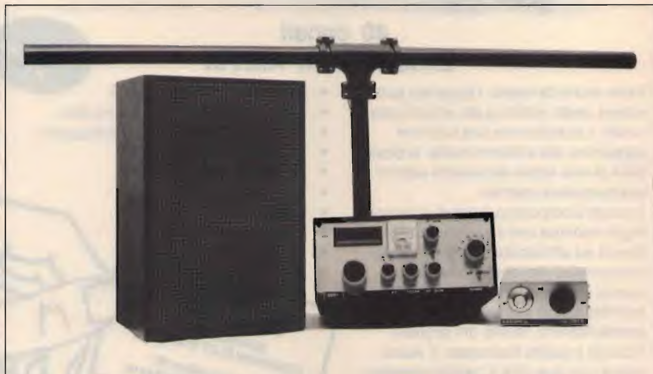
Sistema completo del ricevitore sincrodina per onde lunghe e medie: la control box di comando dell'antenna attiva in ferrite LPF1R; il ricevitore sincrodina "SDR1" e la cassa acustica di tipo attivo utilizzata quale amplificatore di potenza in bassa frequenza che permette di apprezzare totalmente la qualità di riproduzione audio del demodulatore sincrono. Sul fondo domina l'elemento ricevente dell'antenna LPF1R (110 cm), la cui funzione è duplice: sistema ricevente, e di preselezione del segnale ricevuto.
