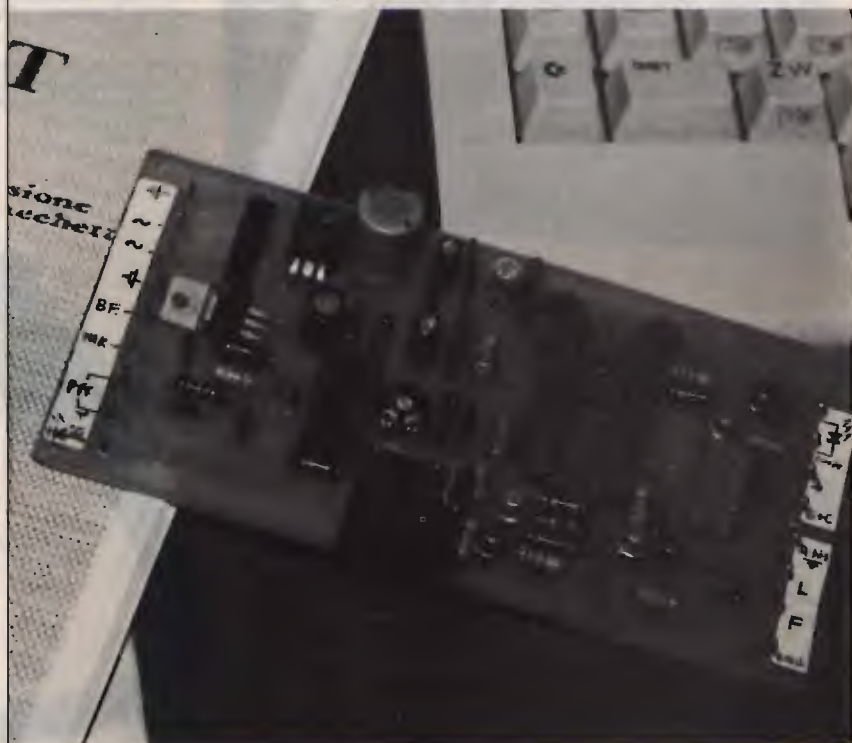
foto 1 Modem Packet non finito (manca l'optoisolatore).
