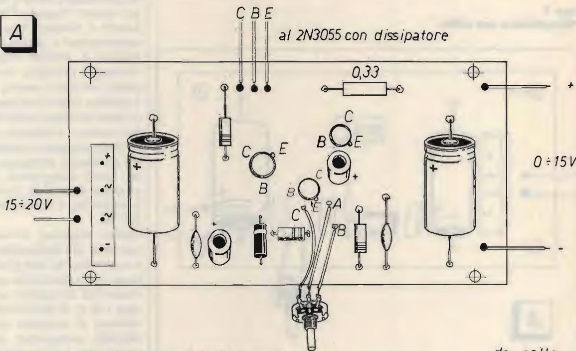
Disposizione componenti visti dal lato rame (trasparenza).
