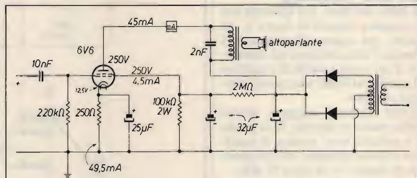
figura 2 Stadio finale di un RX valvolare.
