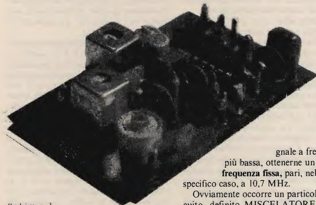
Il telaietto n. 3 a montaggio ultimato.
