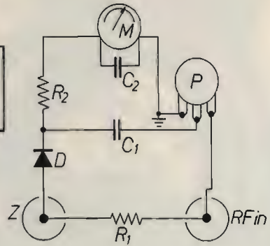
Schema pratico.
