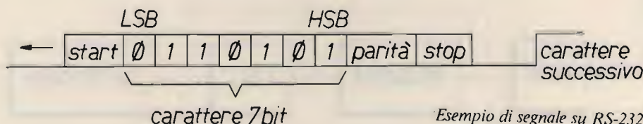
Esempio di segnale su RS-232C
