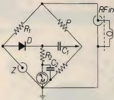
Schema elettrico.
